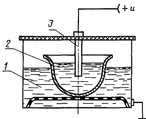
1 - электролит; 2 - корпус каски; 3 - подвижной электрод
