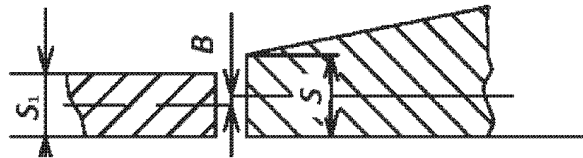
Рисунок 12.2. Смещение кромок листов в стыковых продольных соединениях
