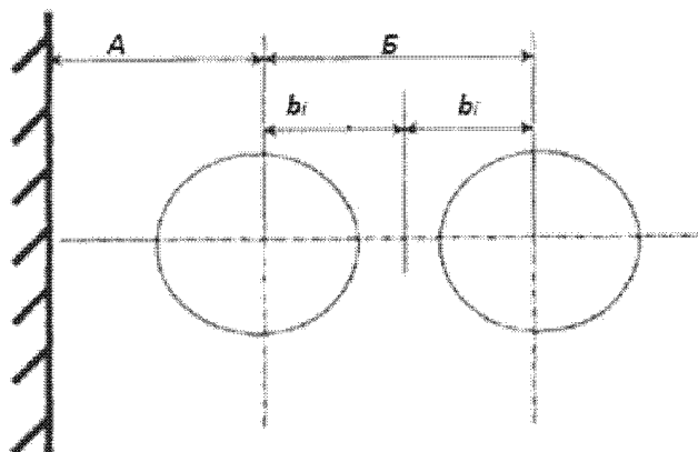
Рисунок 10.1. Расположение трубопроводов
