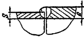
г - соединение без скоса кромок
