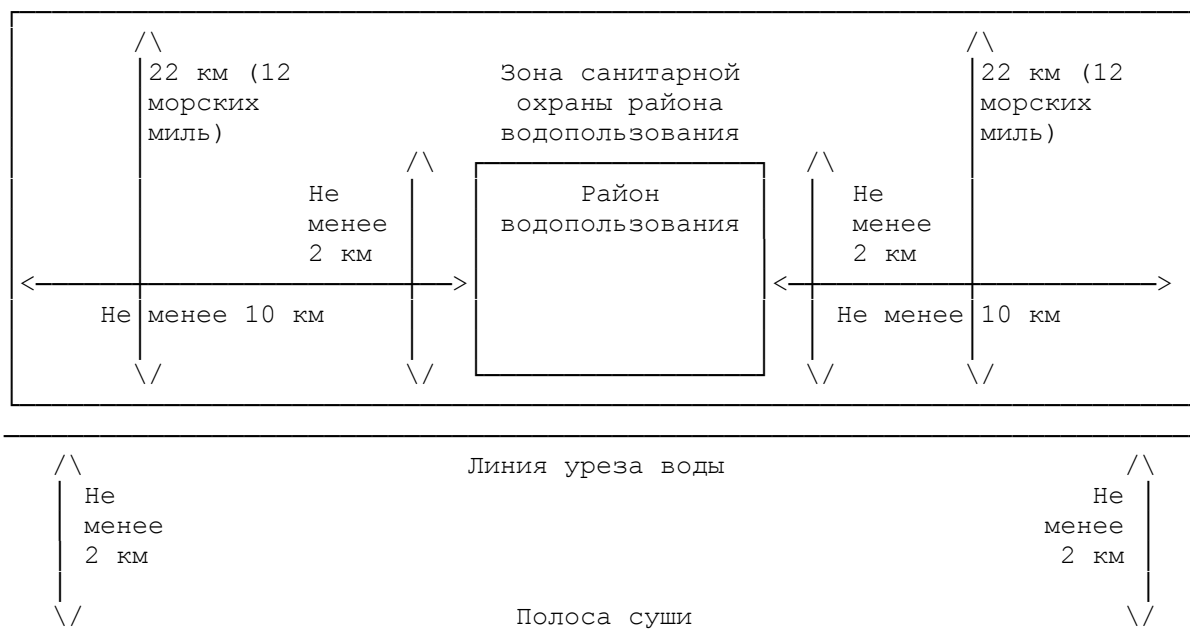
Рисунок 1. Схема охраняемого района
