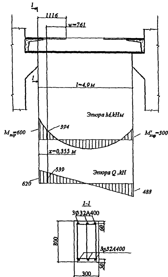
Черт. 3.26. К примеру расчета 21
