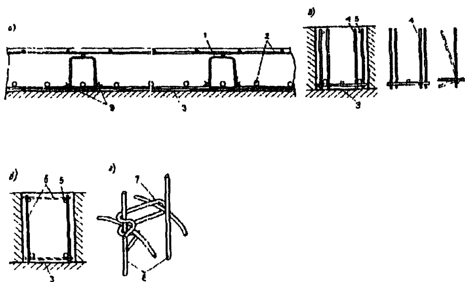
Черт. 5.13. Фиксаторы однократного использования, обеспечивающие требуемое расстояние а - в - между отдельными арматурными изделиями; г - между стержнями; 1 - разделитель из арматурной стали, устанавливаемый между рядами сеток; 2 - фиксатор-подкладка для обеспечения защитного слоя бетона; 3 - удлиненные поперечные стержни каркаса, загибаемые вокруг стержней сетки; 4 - фиксатор для соединения перекрещивающихся стержней (пространственная спираль из пружинной проволоки); 5 - место связи
