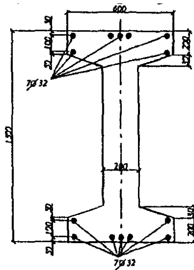
Черт. 3.34. К примерам расчета 28 и 29
