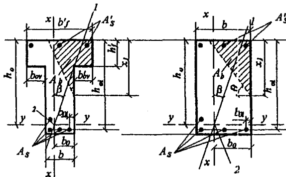
Черт. 3.5 Форма сжатой зоны в поперечном сечении железобетонного элемента, работающего на косой изгиб а - таврового сечения; б - прямоугольного сечения; 1 - плоскость действия изгибающего момента; 2 - центр тяжести сечения растянутой арматуры
