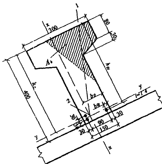
Черт. 3.8. К примеру расчета 10
