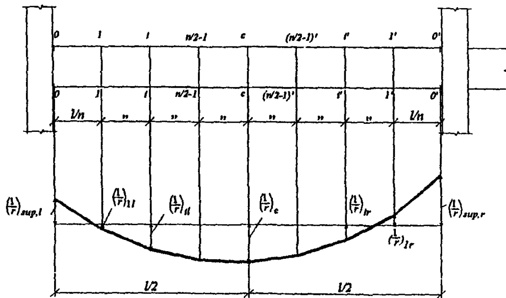
Черт. 4.5. Эпюра кривизны в железобетонном элементе при общем случае определения прогиба
