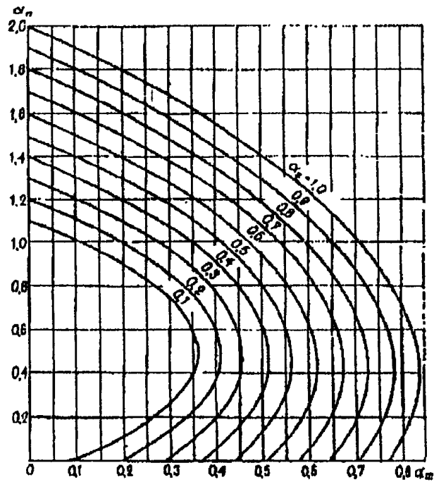
Черт. 3.31. Графики несущей способности внецентренно сжатых элементов кольцевого сечения
