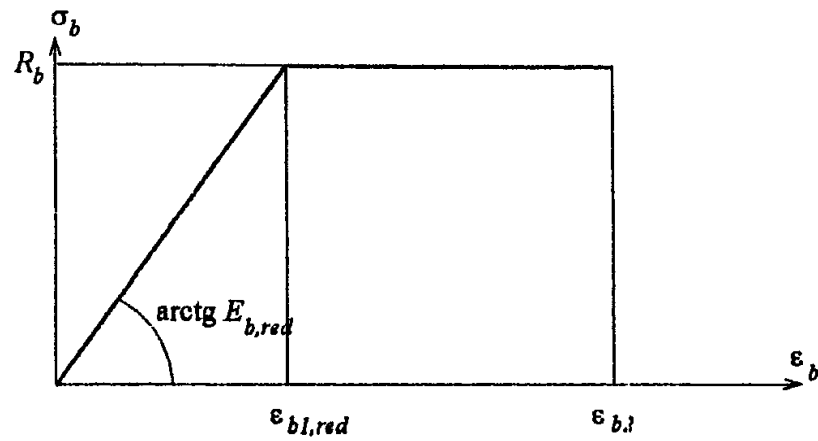
Черт. 3.37. Двухлинейная диаграмма состояния сжатого бетона
