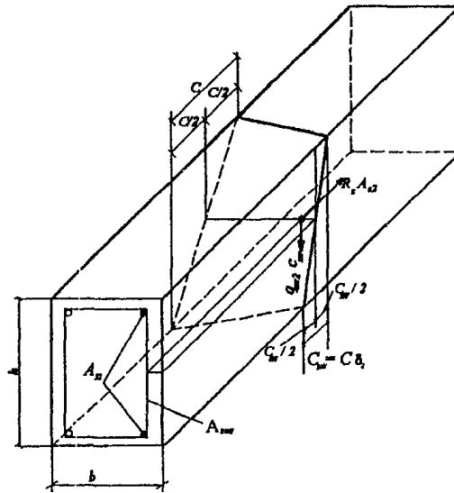
Черт. 3.42. Схемы усилий в пространственных сечениях при расчете на действие крутящего момента и поперечной силы; растянутая арматура у боковой грани элемента
