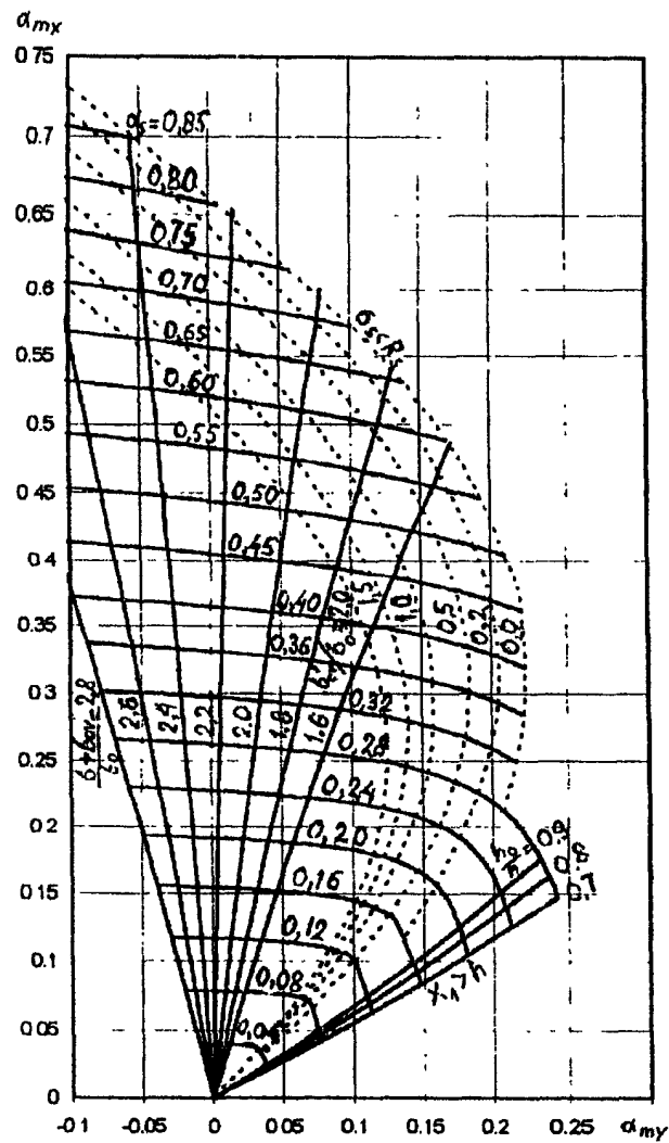
Черт. 3.7. График несущей способности прямоугольного, таврового и Г-образного сечений для элементов, работающих на косои изгиб
