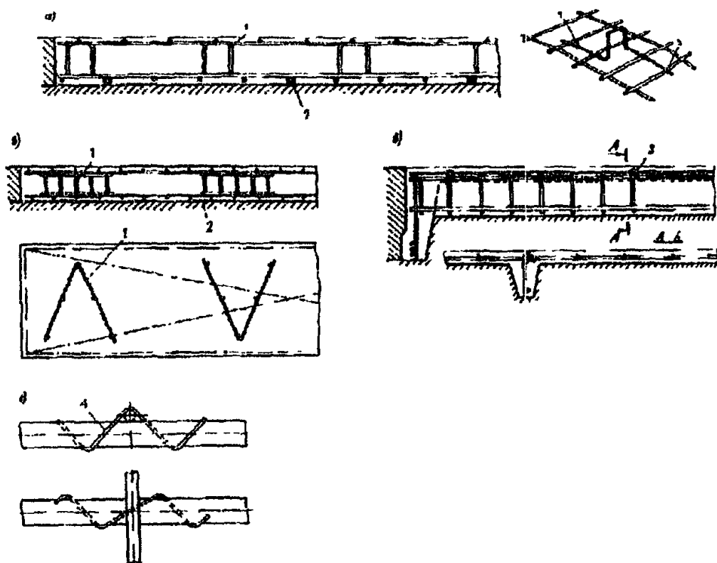
Черт. 5.13. Фиксаторы однократного использования, обеспечивающие требуемое расстояние а - в - между отдельными арматурными изделиями; г - между стержнями; 1 - разделитель из арматурной стали, устанавливаемый между рядами сеток; 2 - фиксатор-подкладка для обеспечения защитного слоя бетона; 3 - удлиненные поперечные стержни каркаса, загибаемые вокруг стержней сетки; 4 - фиксатор для соединения перекрещивающихся стержней (пространственная спираль из пружинной проволоки); 5 - место связи
