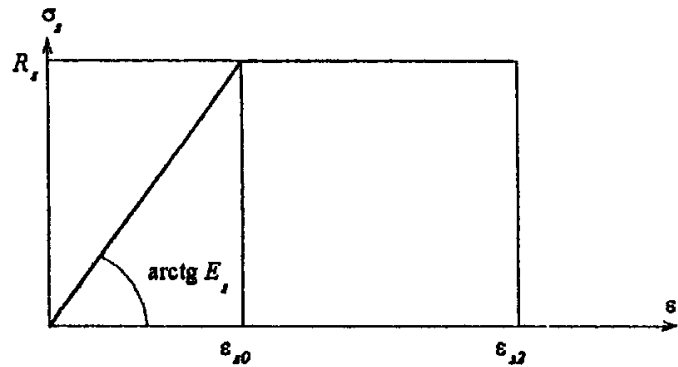
Черт. 3.38. Диаграмма состояния растянутой арматуры
