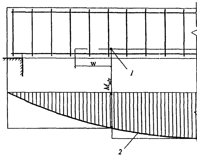
Черт. 3.20. Обрыв растянутых стержней в пролете
