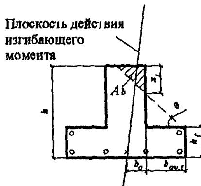
Черт. 3.6. Тавровое сечение со сжатой зоной, заходящей в наименее растянутый свес полки
