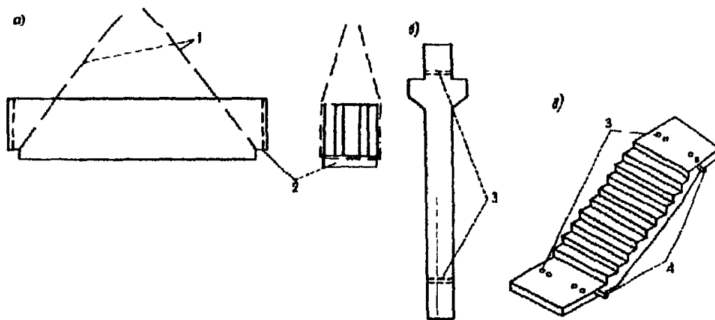
Черт. 5.9. Примеры строповочных устройств без петель
