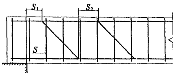
Черт. 3.16. Расстояния между хомутами, опорой и отгибами
