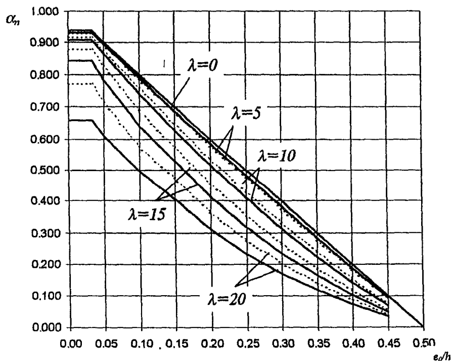
Черт. 3.2. График несущей способности внецентренно сжатых бетонных элементов
