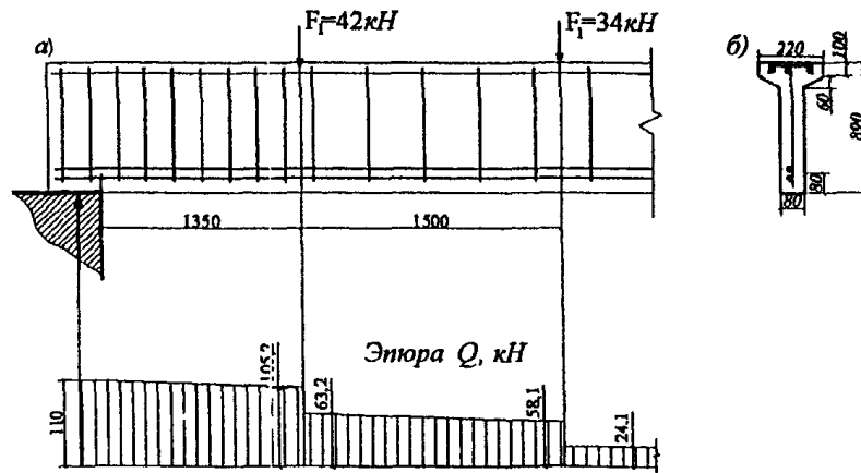
Черт. 3.22. К примеру расчета 15
