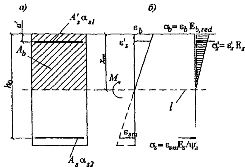
Черт. 4.7. Приведенное поперечное сечение (а) и схема напряженно-деформированного состояния изгибаемого элемента с трещинами при расчете его по деформациям ( \delta )
