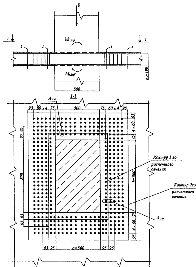
Черт. 3.50. К примеру расчета 40
