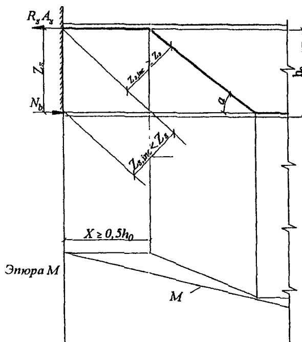
Черт. 3.21. К определению места отгиба продольной растянутой арматуры
