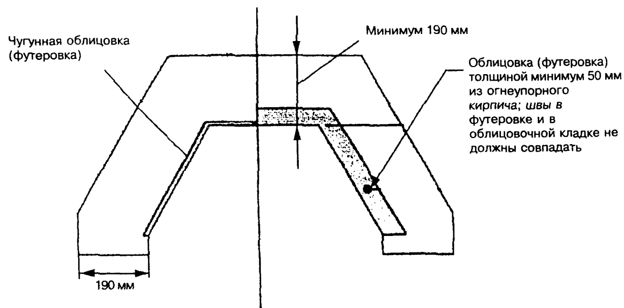
Рисунок 7.5. Футеровка камина
