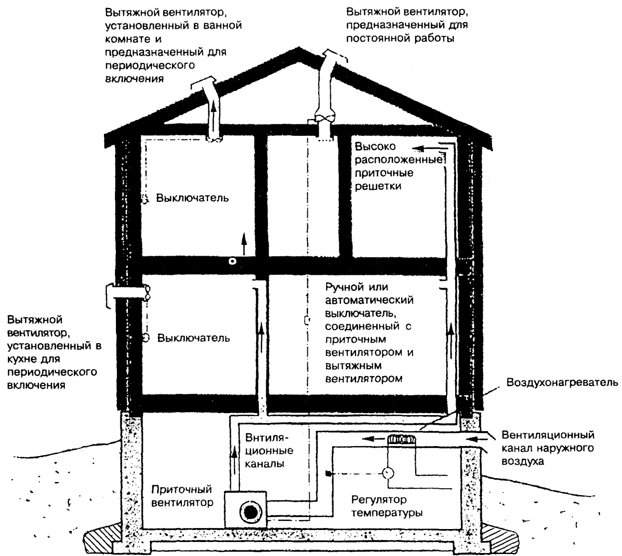
Рисунок 7.2. Система воздушного отопления с принудительной циркуляцией воздуха,
