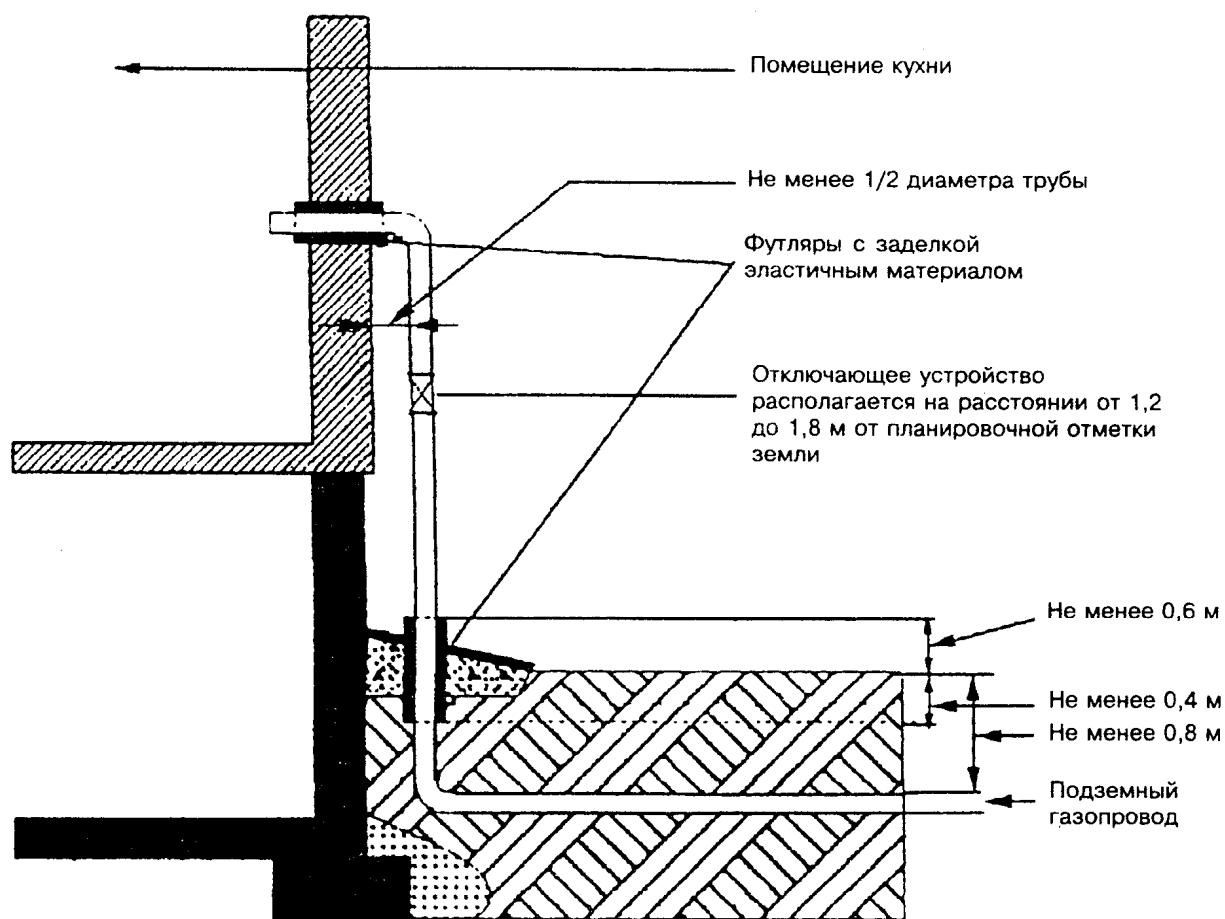
Рисунок 9.1. Газовый ввод
