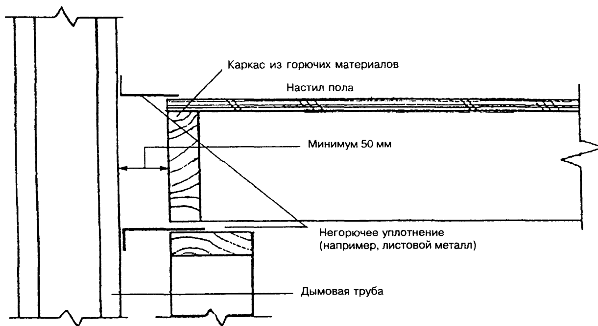
Рисунок 7.8. Расстояние от дымовой трубы до строительных конструкций
