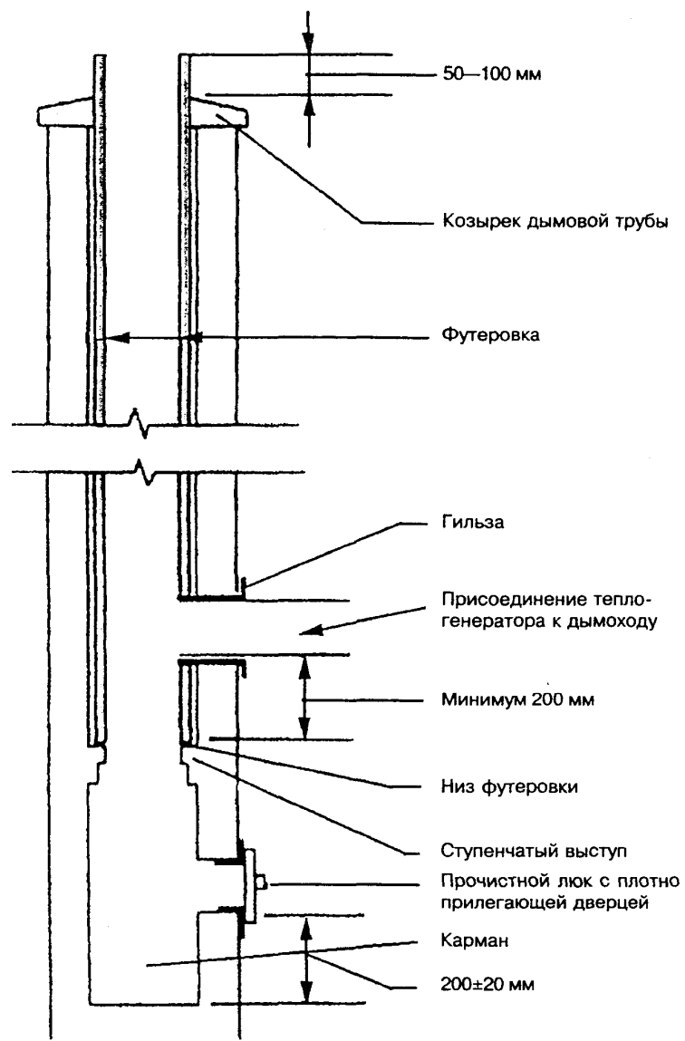
Рисунок 7.6. Облицовка дымохода
