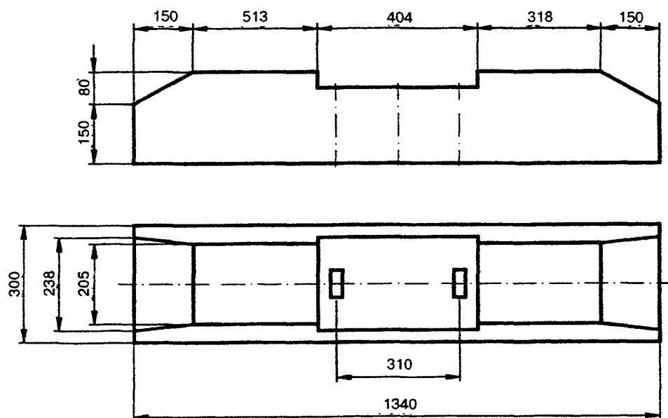
Б2. Железобетонная полупала типа ПШН4-13-325-1
