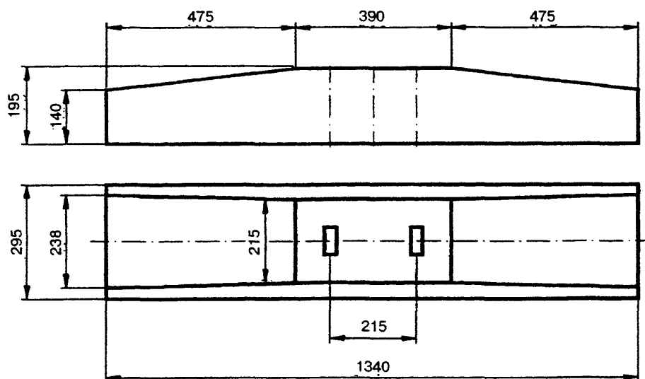
Б2. Железобетонная полупала типа ПШН4-13-325-1
