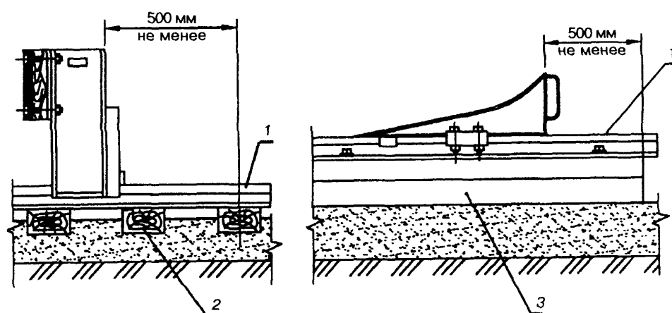
г) установка тупиковых упоров на рельсовой нити
