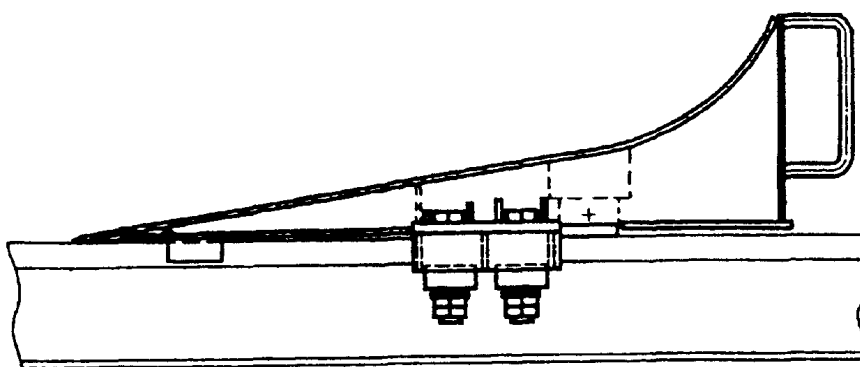
Г.8. КОНСТРУКЦИИ ТУПИКОВЫХ УПОРОВ И ИХ УСТАНОВКА НА КРАНОВОМ ПУТИ
