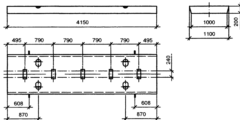
Б4. Железобетонная плита
