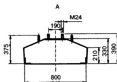
Б4. Железобетонная плита
