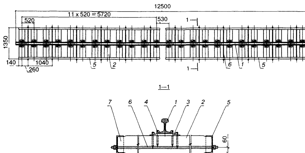
Г.14. ИНВЕНТАРНЫЕ ДЕРЕВОМЕТАЛЛИЧЕСКИЕ СЕКЦИИ (с использованием деревянных полушпал)
