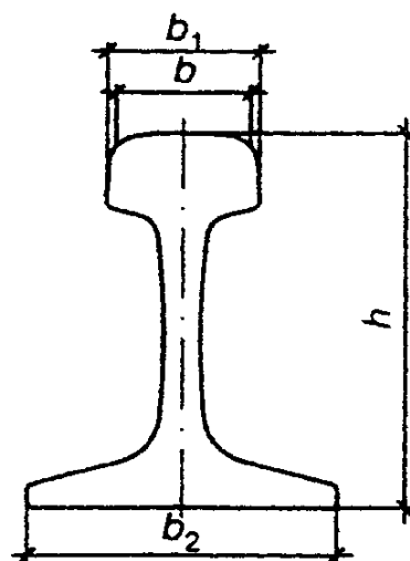
Г.4. КОНСТРУКЦИЯ И ОСНОВНЫЕ ХАРАКТЕРИСТИКИ РЕЛЬСОВ
