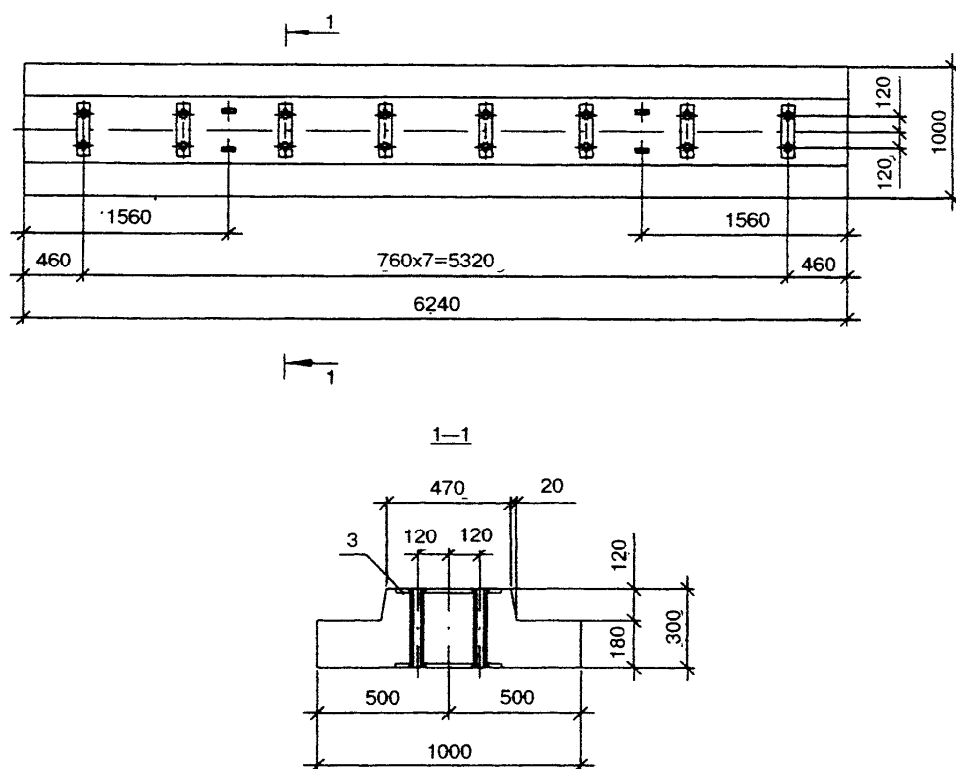
Г.4. КОНСТРУКЦИЯ И ОСНОВНЫЕ ХАРАКТЕРИСТИКИ РЕЛЬСОВ
