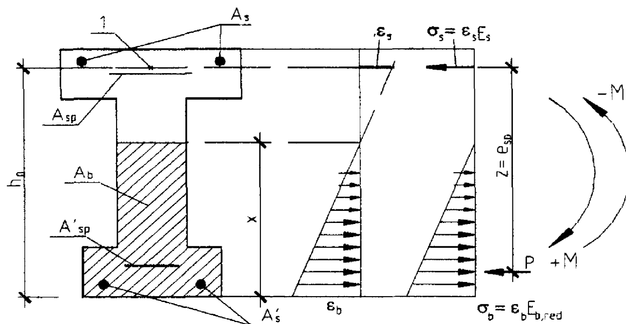
Черт. 4.5. Схемы усилий и напряженно-деформированного состояния сечения с трещиной в стадии изготовления
