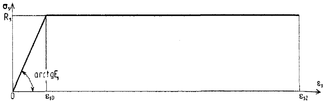
Черт. 3.11. Двухлинейная диаграмма состояния арматуры с физическим пределом текучести
