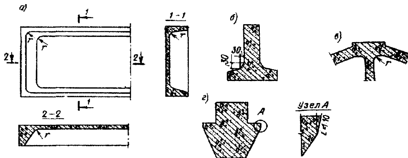
Черт. 5.6. Закругления и фаски
