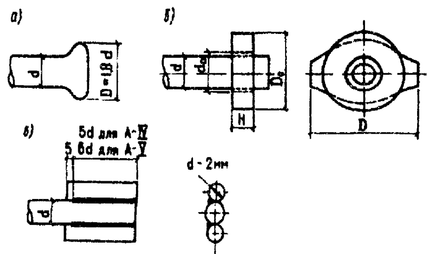
Черт. 5.5. Временные технологические анкера на напрягаемой стержневой арматуре
