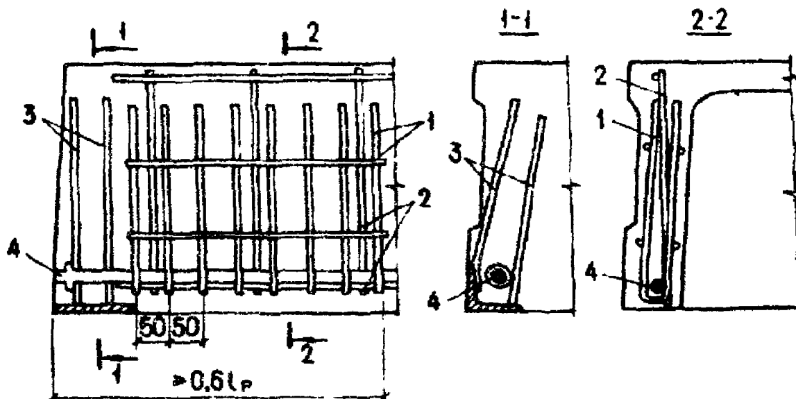
Черт. 5.4. Армирование конца ребра плиты перекрытия
