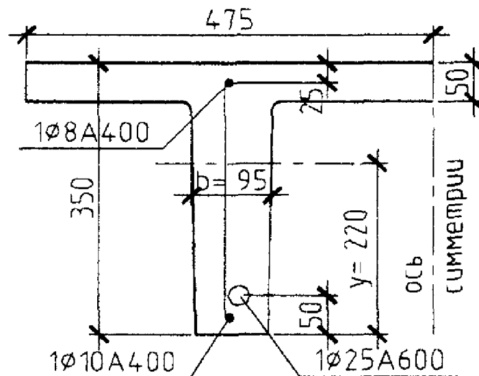
Черт. 4.7. К примерам расчета 19, 20 и 21
