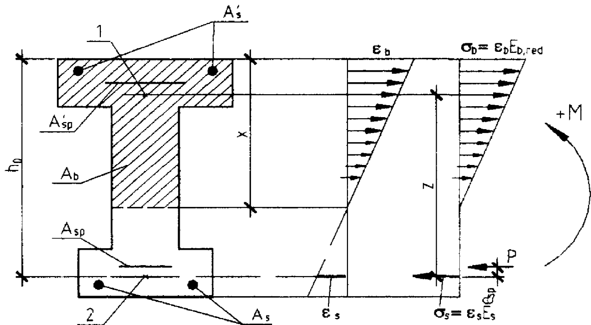
Черт. 4.4. Схемы усилий и напряженно-деформированного состояния сечения с трещиной в стадии эксплуатации при расчете по раскрытию трещин
