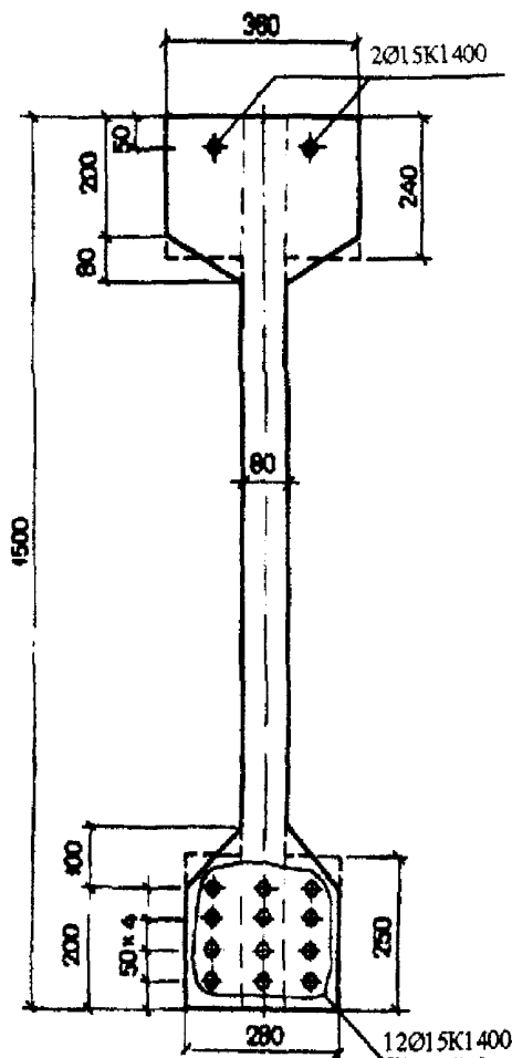
Черт. 2.3. К примеру расчета 2
