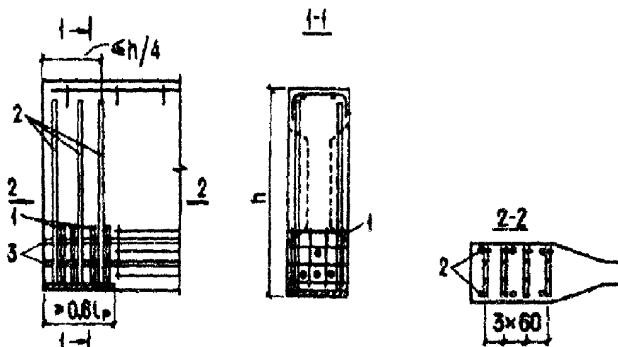
Черт. 5.2. Армирование конца предварительно напряженной балки
