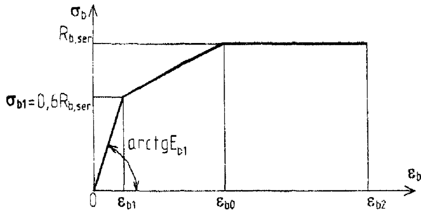
Черт. 4.11. Трехлинейная диаграмма состояния сжатого бетона при расчетах по 2-й группе предельных состояний
