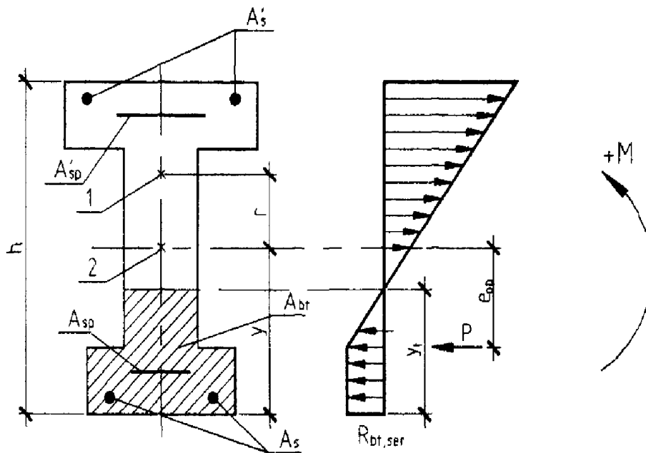
Черт. 4.1. Схема усилий и эпюра напряжений в поперечном сечении элемента при расчете по образованию трещин в стадии эксплуатации
