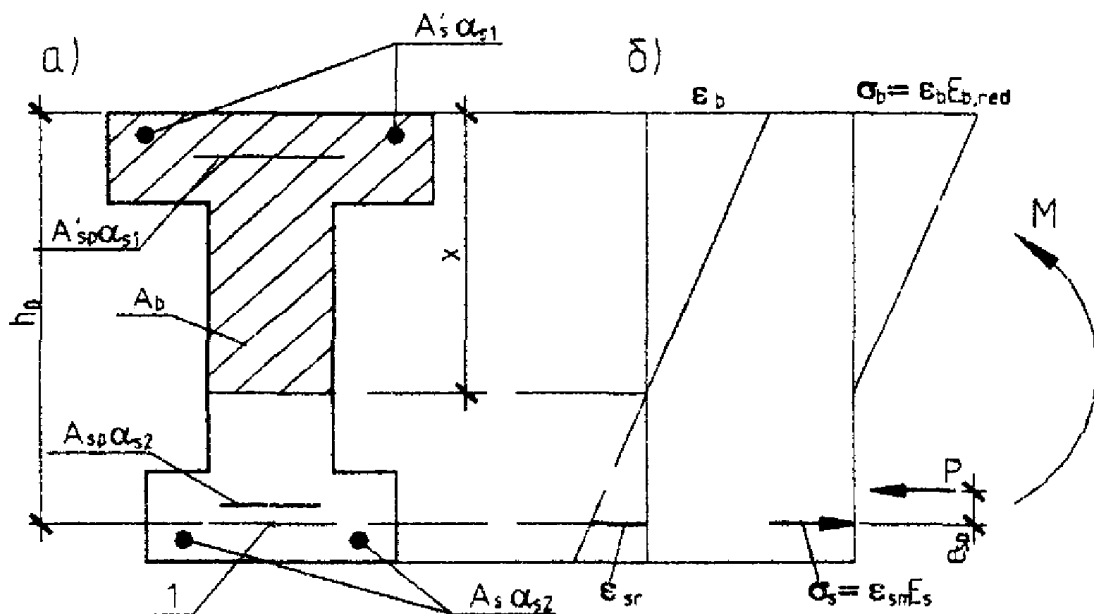
Черт. 4.10. Приведенное поперечное сечение (а) и схема напряженно деформированного состояния изгибаемого предварительно напряженного элемента с трещинами (б) при расчете его по деформациям
