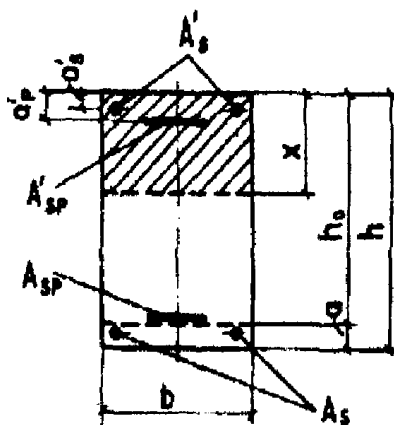
Черт. 3.1. Поперечное прямоугольное сечение изгибаемого железобетонного элемента
