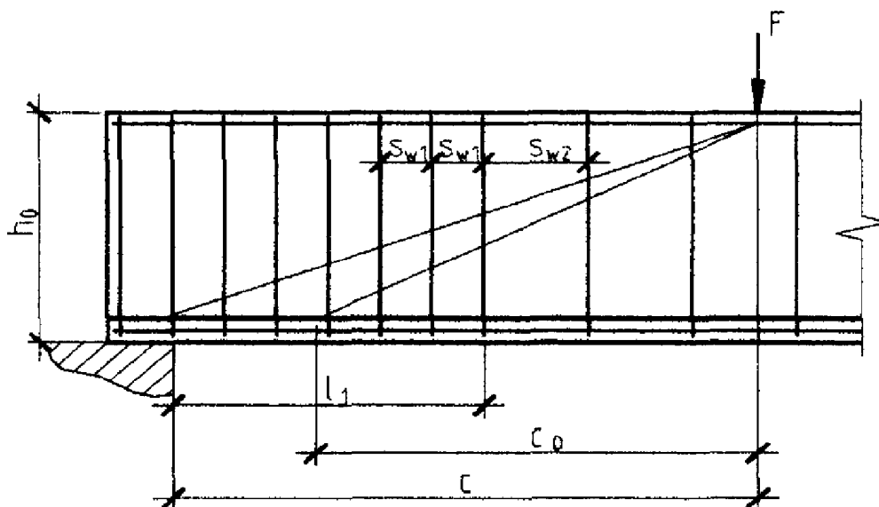
Черт. 3.17. Изменение интенсивности хомутов в пределах наклонного сечения
