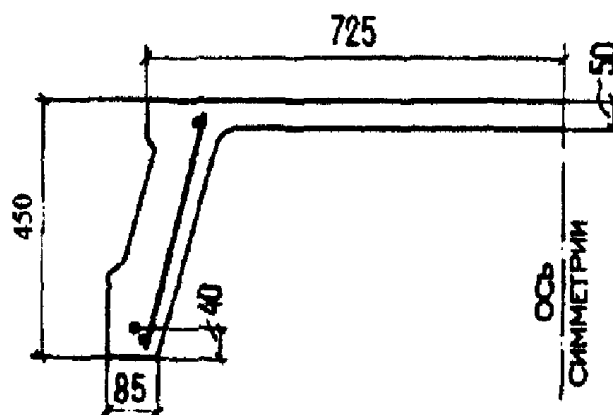
Черт. 3.22. К примеру расчета 11
