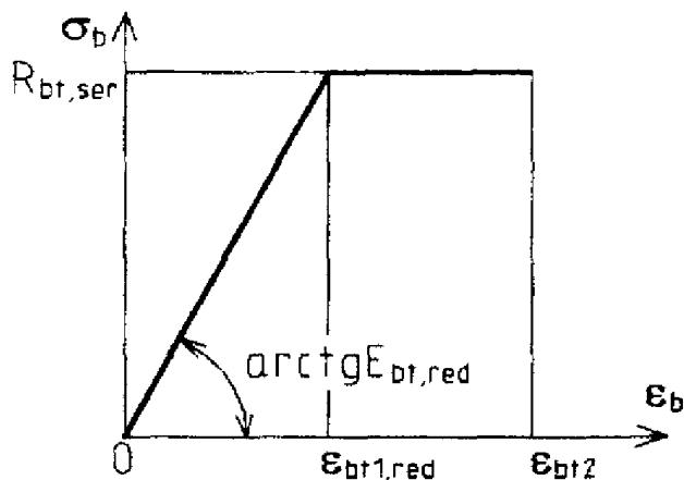
Черт. 4.3. Двухлинейная диаграмма состояния растянутого бетона
