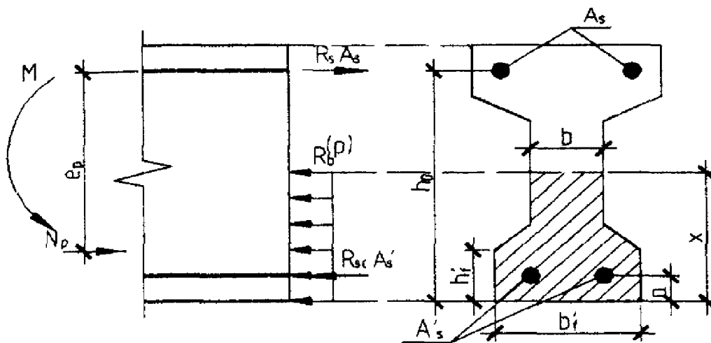
Черт. 3.7. Схема усилий в поперечном сечении железобетонного элемента с полкой в сжатой зоне в стадии предварительного обжатия
