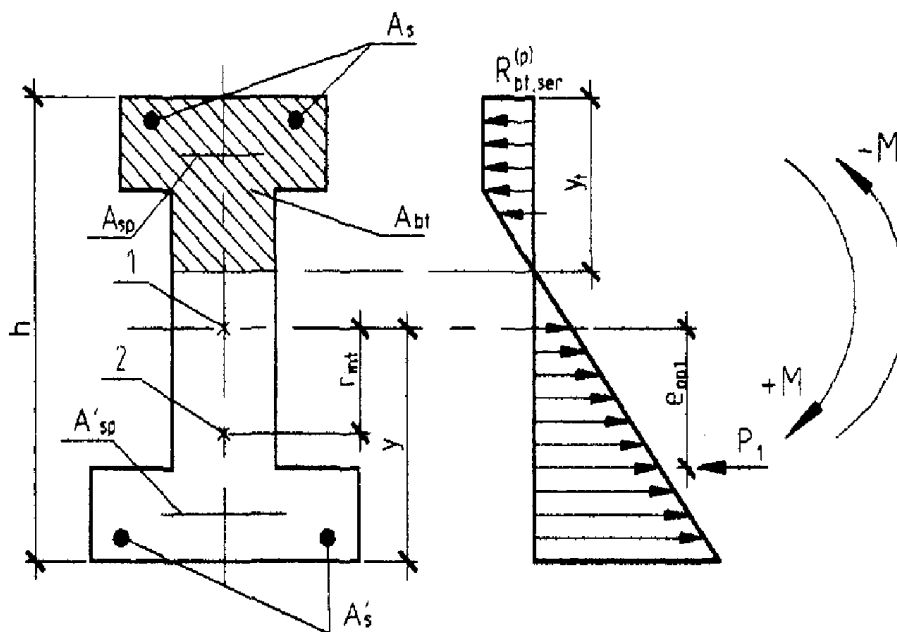
Черт. 4.2. Схема усилий и эпюра напряжений в поперечном
