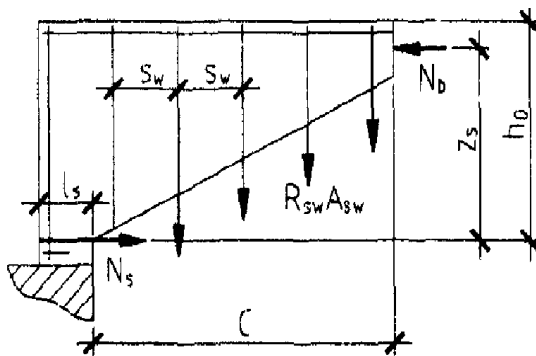
Черт. 3.20. Схема усилий в наклонном сечении при расчете по изгибающему моменту
