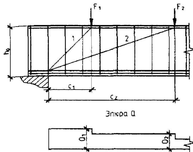
Черт. 3.16. Расположение расчетных наклонных сечений при сосредоточенных силах
