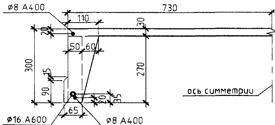
Черт. 2.2. К примеру расчета 1
