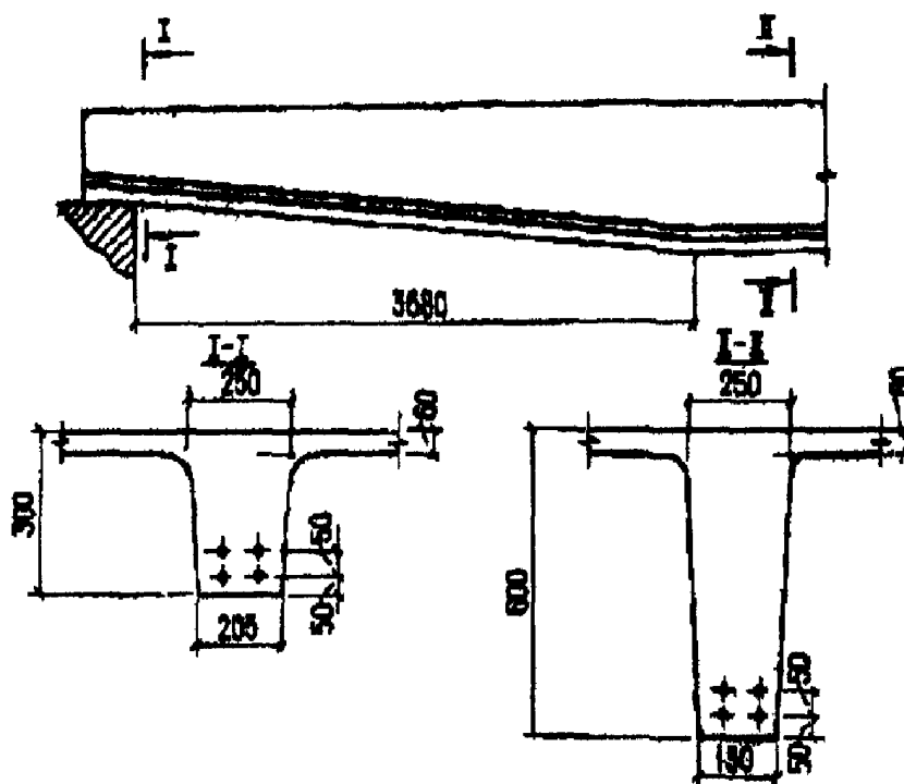
Черт. 3.24. К примеру расчета 14
