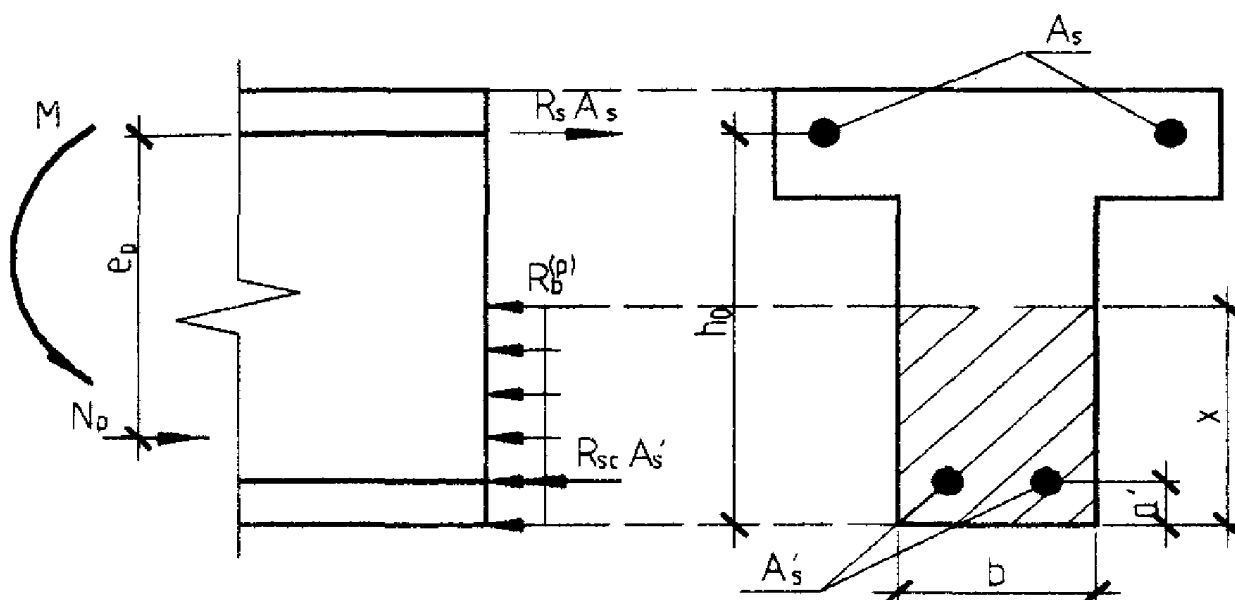
Черт. 3.6. Схема усилий в поперечном сечении железобетонного элемента с прямоугольной сжатой зоной в стадии предварительного обжатия
