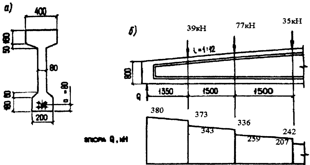
Черт. 3.25. К примеру расчета 15
