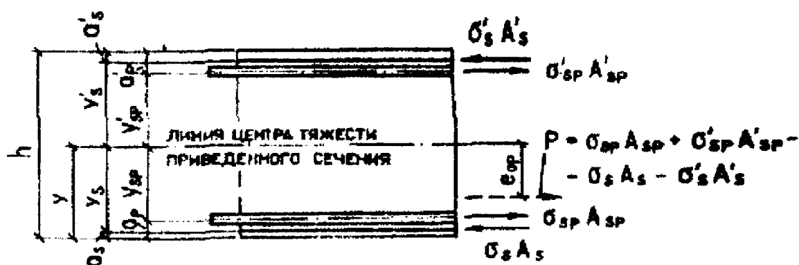
Черт. 2.1. Схема усилий предварительного напряжения арматуры в поперечном сечении железобетонного элемента
