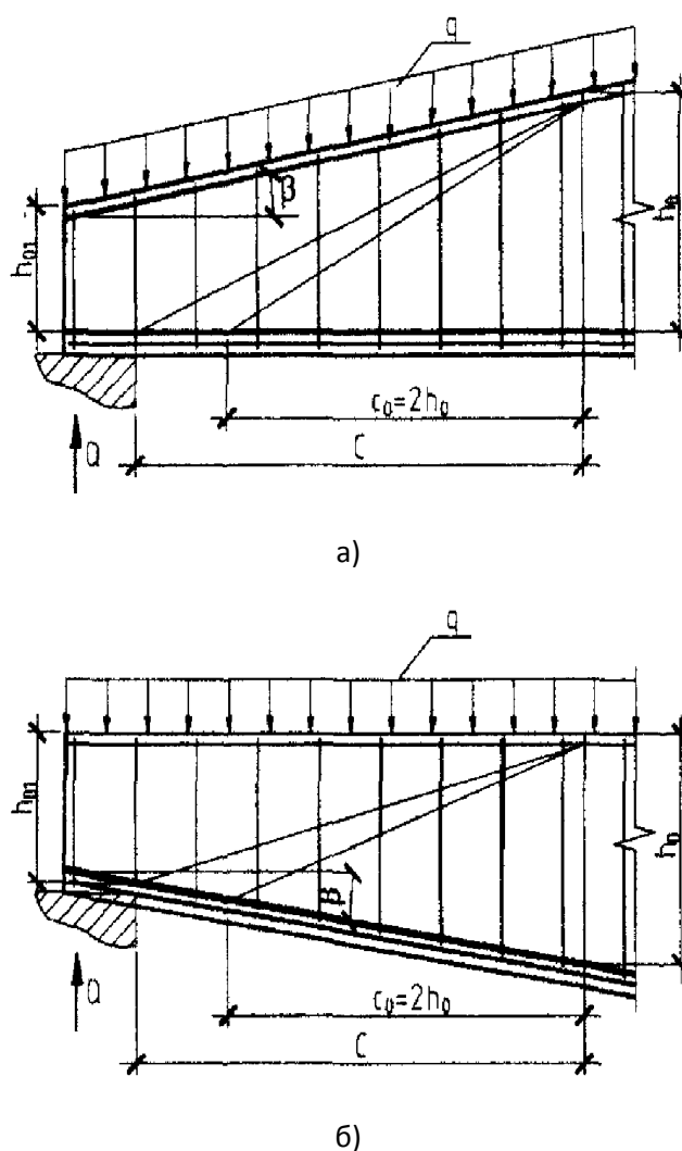
Черт. 3.18. Наклонные сечения балок с переменной высотой сечения
