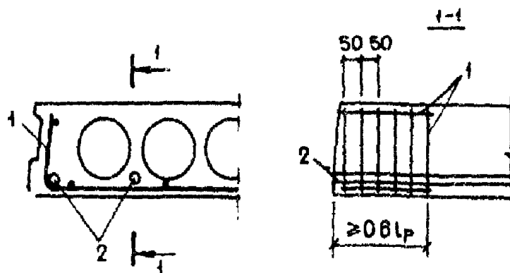
Черт. 5.3. Армирование конца многопустотного настила
