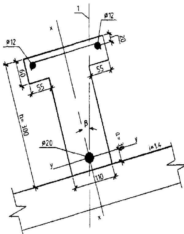
Черт. 3.5. К примеру расчета 9
