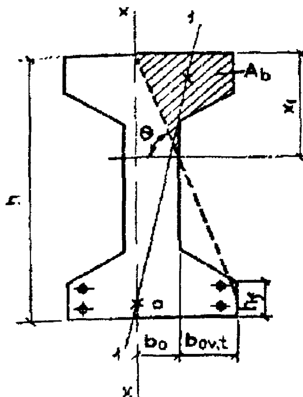
Черт. 3.4. Двутавровое сечение со сжатой зоной, заходящей в наименее растянутый свес полки
