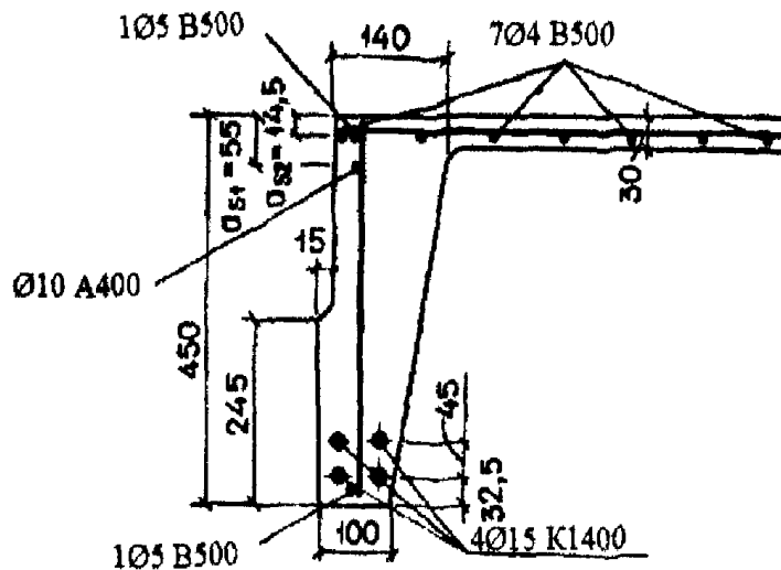
Черт. 3.9. К примеру расчета 10
