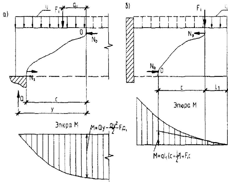
Черт. 3.21. Определение расчетного значения момента при расчете наклонного сечения
