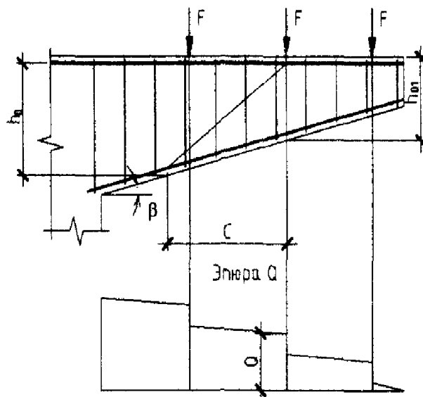
Черт. 3.19. Наклонное сечение консоли с переменной высотой сечения
