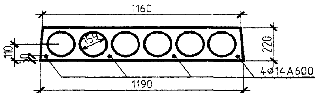
Черт. 3.26. К примеру расчета 16
