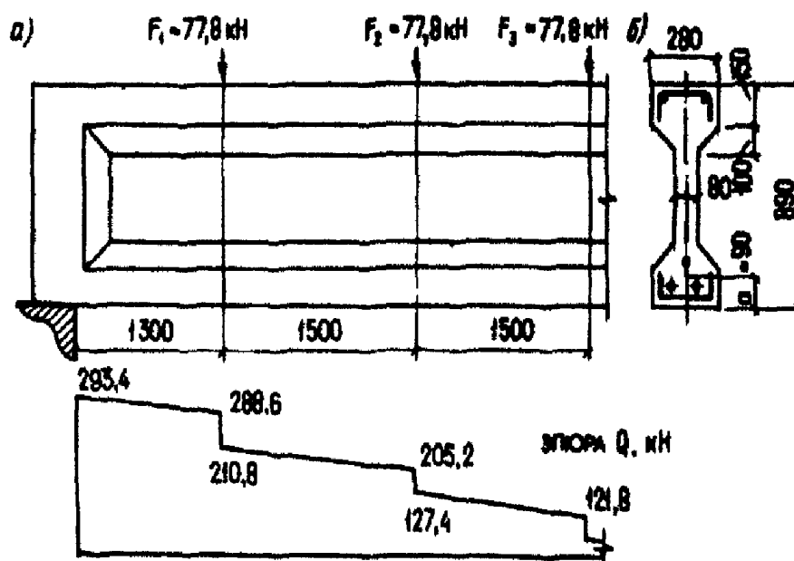
Черт. 3.23. К примеру расчета 13
