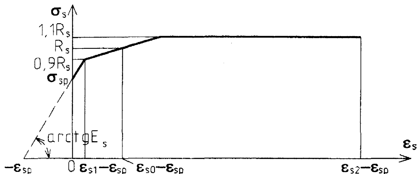
Черт. 3.13. Трехлинейная диаграмма состояния арматуры с условным пределом текучести при учете предварительного напряжения (здесь \varepsilon_s - деформация арматуры от внешней нагрузки)
