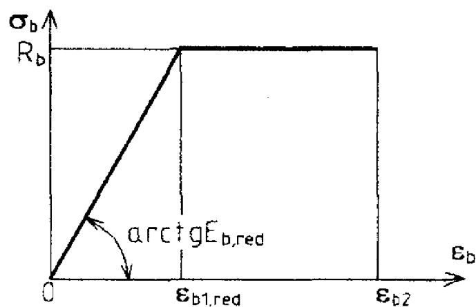
Черт. 3.10. Двухлинейная диаграмма состояния сжатого бетона
