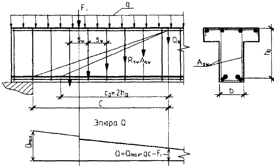
Черт. 3.15. Схема усилий в наклонном сечении элемента, армированного хомутами, при расчете на действие поперечной силы
