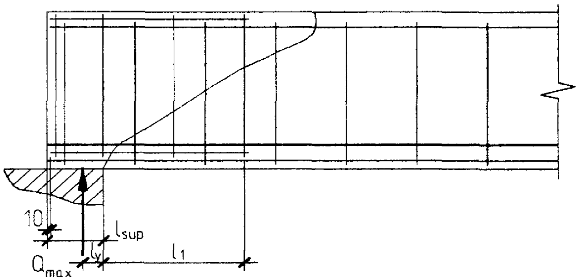
Черт. 3.27. К примеру расчета 17
