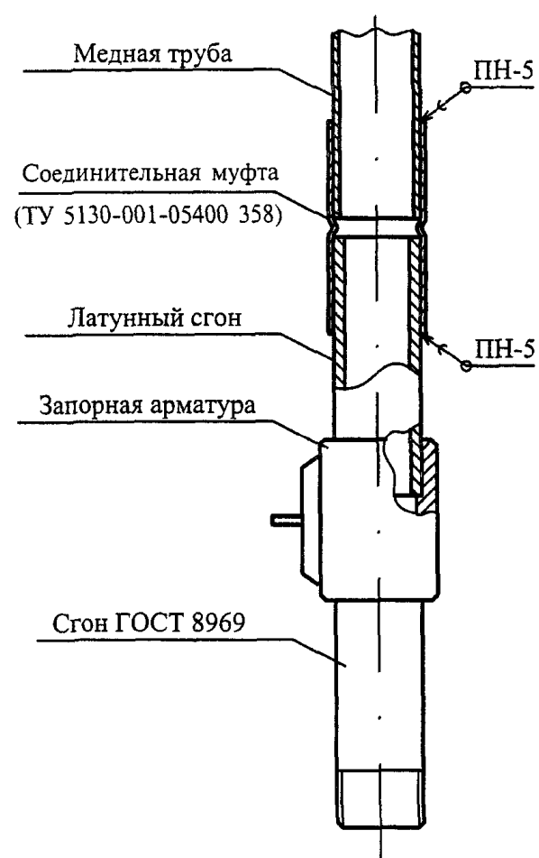
Рисунок 6. Присоединение запорной арматуры к медному газопроводу
