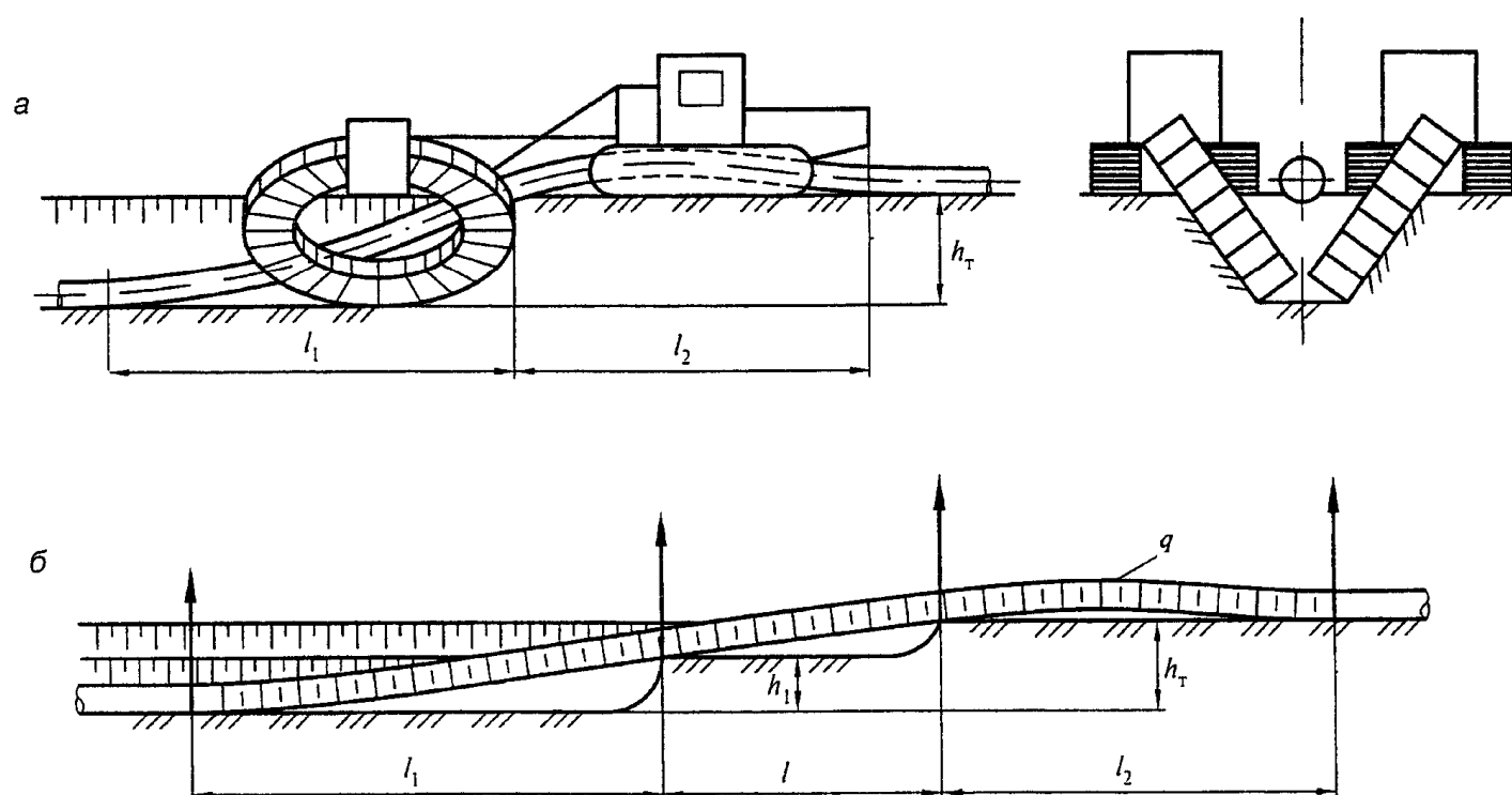
Рисунок 23. Укладка газопровода методом "подкопа"
