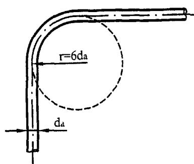
Рисунок 13. Холодная гибка медной трубы
