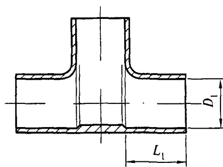
Рисунок Д.5. Тройник равнопроходный
