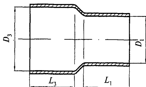
Рисунок Д.3. Переход
