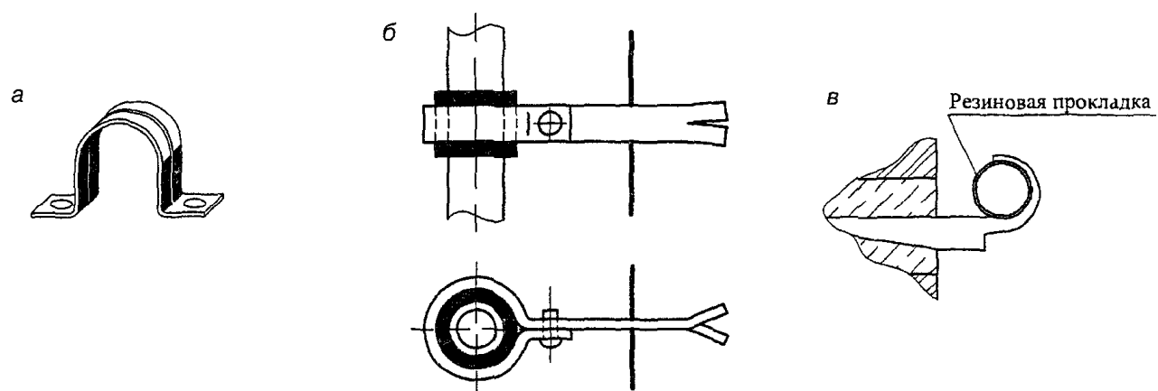
Рисунок 5. Опоры для крепления медных газопроводов
