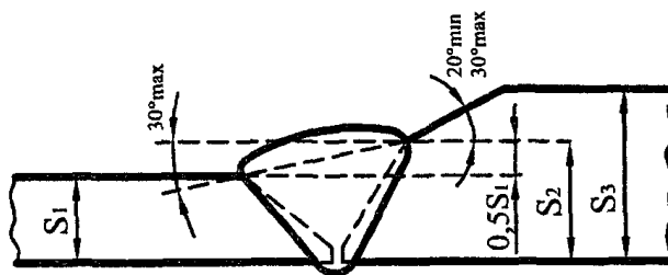
Рисунок 10. Обработка свариваемых торцов труб
