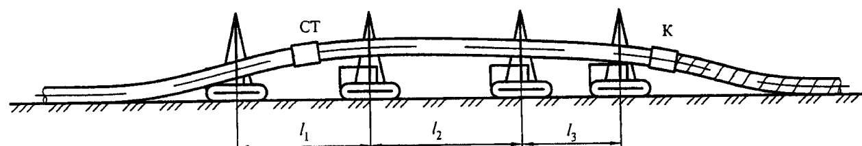
Рисунок 18. Схема расстановки трубоукладчиков для укладки плети газопровода при использовании комбайна для очистки и изоляции труб диаметром: а - 500 мм и менее; б - 700 - 1000 мм; в - 1000 - 1200 мм
