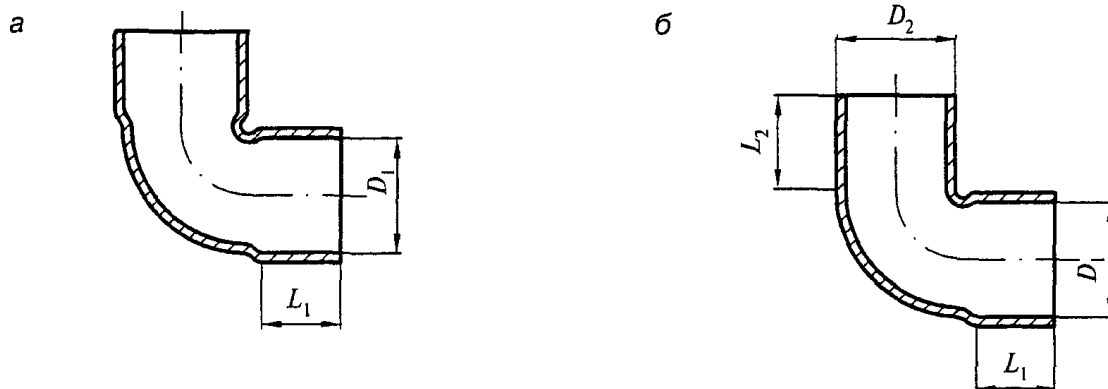
Рисунок Д.4. Отводы
