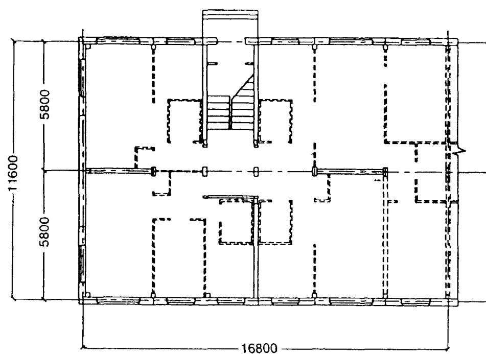
СХЕМА ОРГАНИЗАЦИИ БЛОКА ОБСЛУЖИВАНИЯ В СЕКЦИИ СОЦИАЛЬНОГО ЖИЛЬЯ
