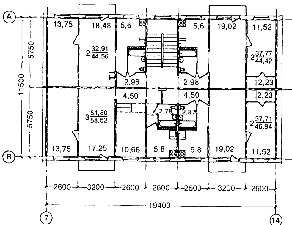
План типового этажа рядовой секции 2-2-2-3
