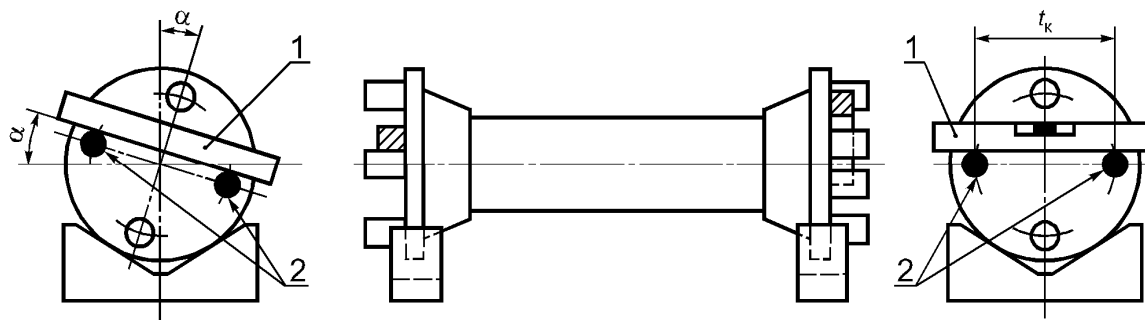
1 - пузырьковый уровень; 2 - центровочные штыри
