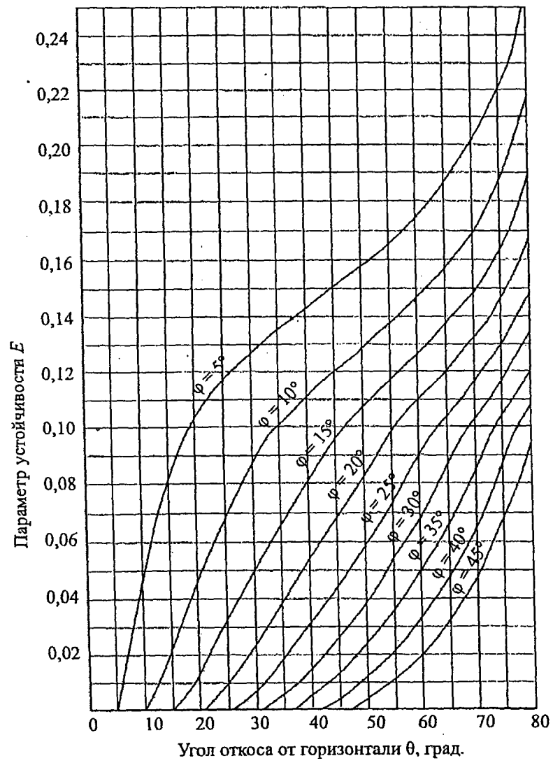
Рисунок В.1. Графики для определения крутизны откоса при K = 0
