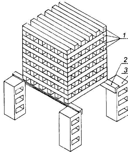
1 - деревянные бруски; 2 - стальной уголок; 3 - бетонный (металлический) блок
