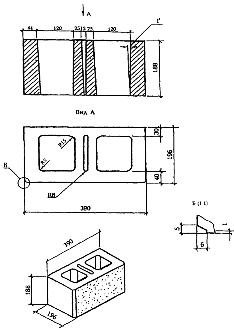
Рисунок Б.12. Камень лицевой декоративный угловой
