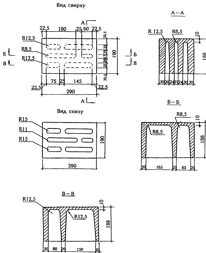
Рисунок Б.3. Камень дополнительный стеновой рядовой (трехчетвертной)
