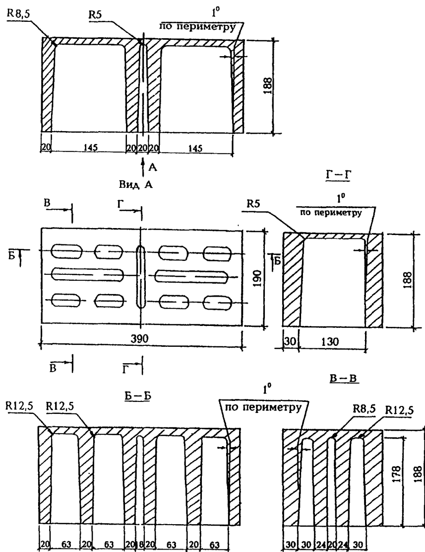
Рисунок Б.2. Камень стеновой рядовой
