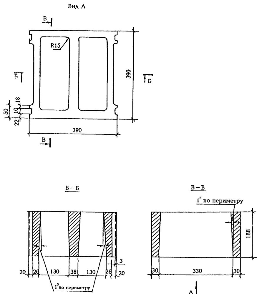
Рисунок Б.21. Камень для вентиляционных каналов
