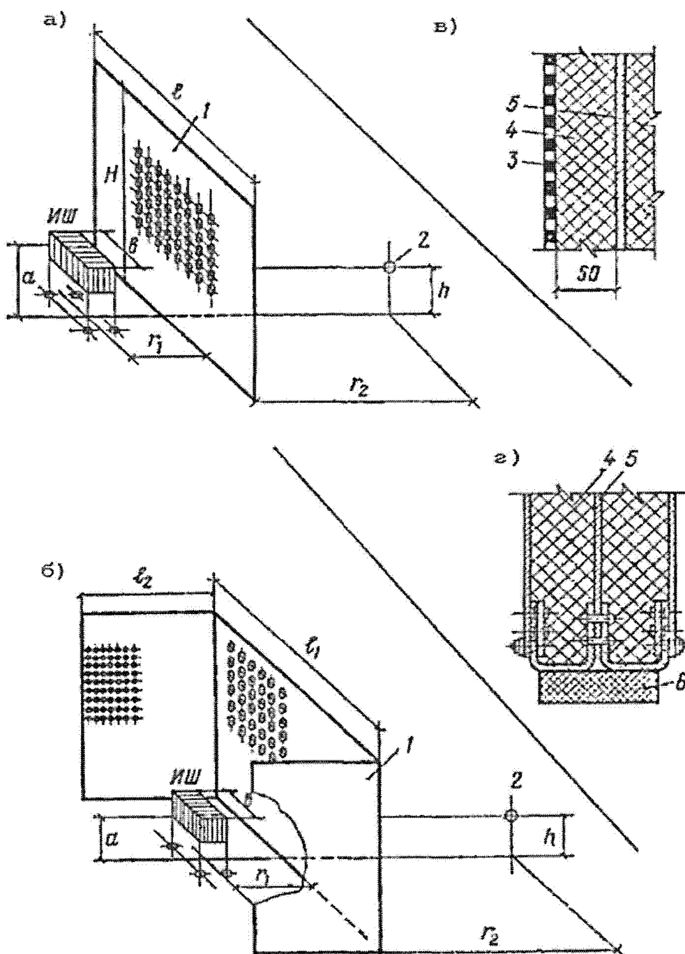
а), б) - формы экрана; в) - конструкция панели экрана; г) - конструкция основания экрана; ИШ - источник шума; 1 - экран; 2 - расчетная точка; 3 - перфорированный лист; 4 - звукопоглотитель;
