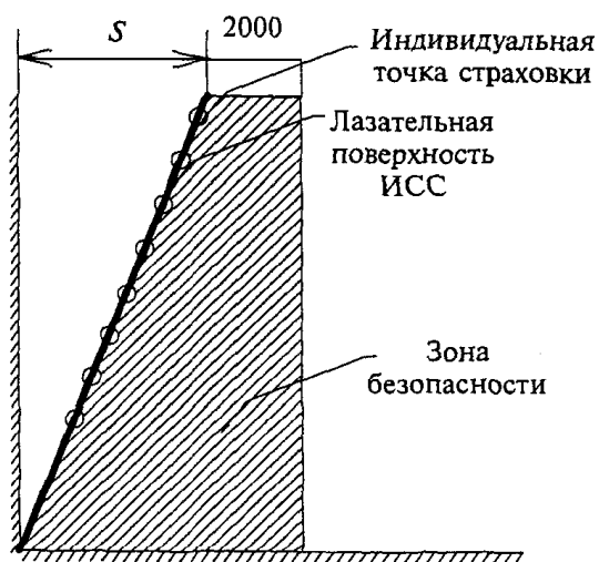
Схема 4.3. Расчет зоны безопасности
