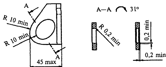
Рисунок Д.2. Выступающая часть индивидуальной страховочной точки
