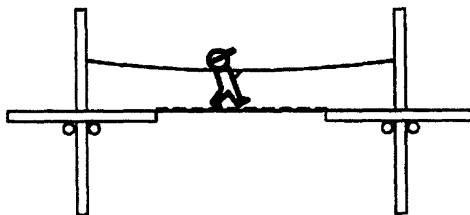
Подвесной мост "Зигзаг" без перил
