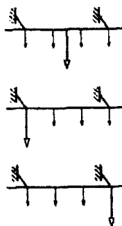
Рисунок Д.4. Размещение расчетных нагрузок на коллективной верхней страховке
