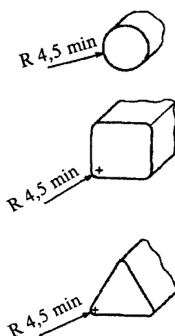
Рисунок Д.3. Скругление краев элементов для крепления веревок (мм)
