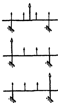
Рисунок Д.5. Размещение нагрузок на коллективных страховочных системах с наземным креплением
