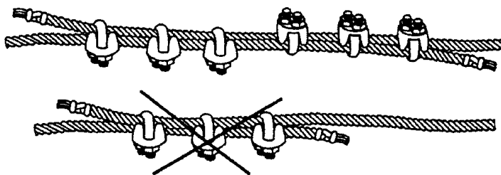
Рисунок В.4. Размещение захватов проволочного каната
