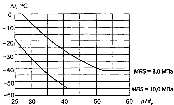
Рисунок 6. Максимально допустимый отрицательный температурный перепад в зависимости от отношения радиуса упругого изгиба к наружному диаметру газопровода при температуре эксплуатации 0 °С и рабочем давлении 0,3 МПа для SDR 17,6 и различных MRS
