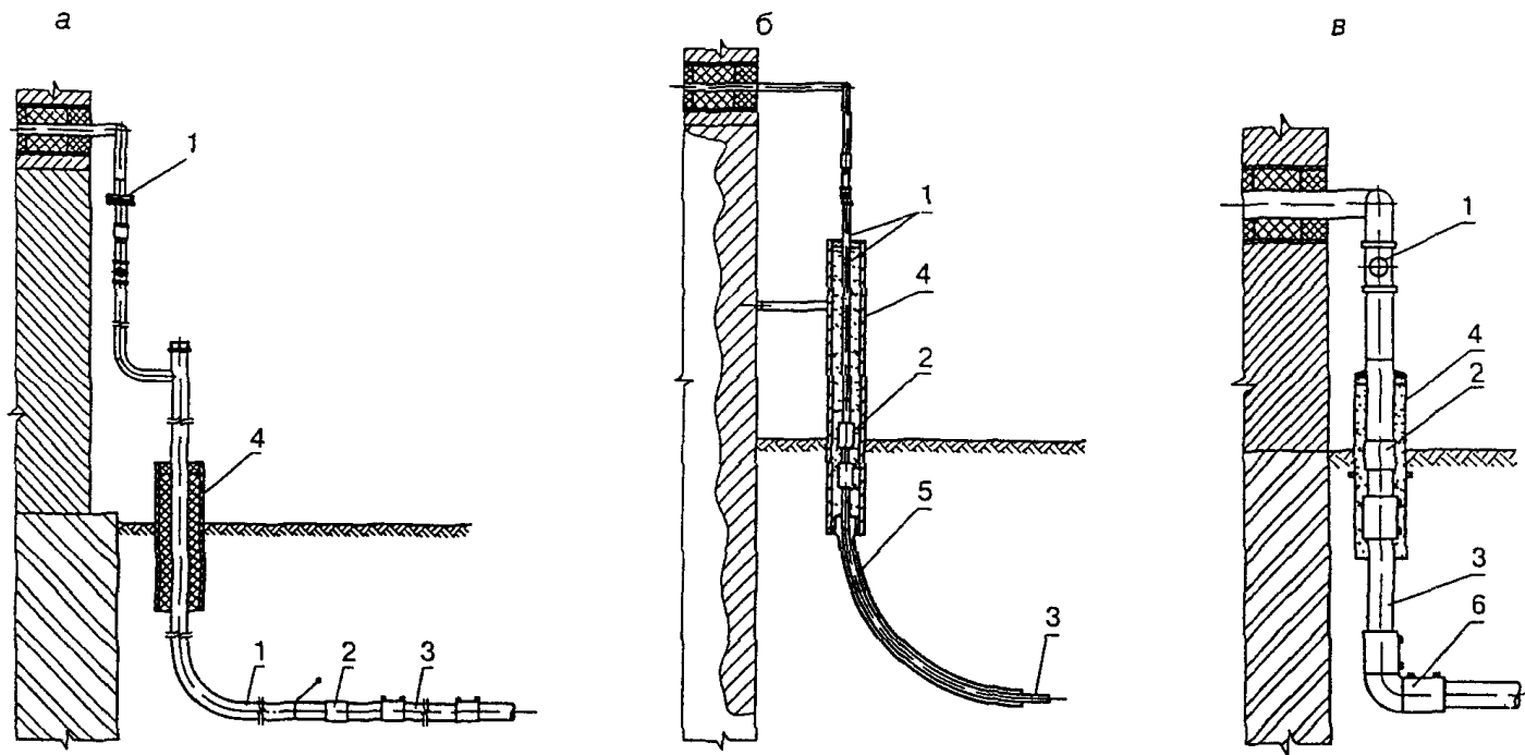
а - стальной цокольный ввод; б - полиэтиленовый ввод, выполненный свободным изгибом трубы; в - полиэтиленовый ввод, выполненный при помощи отвода с ЗН 1 - стальной участок цокольного ввода; 2 - переход "сталь - полиэтилен"; 3 - полиэтиленовый газопровод; 4 - футляр; 5 - полиэтиленовый футляр изогнутый; 6 - отвод с ЗН; 7 - электроизолирующее устройство
