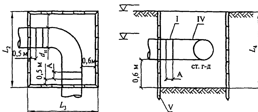
Рисунок Л.3. Вставка отвода
