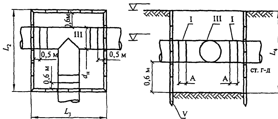
Рисунок Л.2. Вставка тройника
