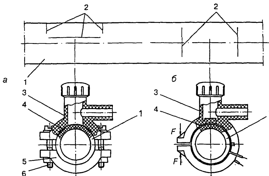
а - седловой отвод с закладным нагревателем; б - отвод с разрезной муфтой с закладным нагревателем; 1 - труба; 2 - метки посадки отводов и механической обработки поверхности трубы; 3 - отвод; 4 - закладной нагреватель; 5 - полухомут; 6 - винты крепления; F - усилие прижатия отвода при сборке и сварке
