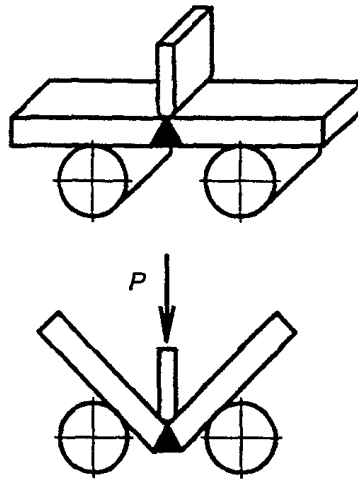
Рисунок Ф.1. Схема испытания на статический изгиб
