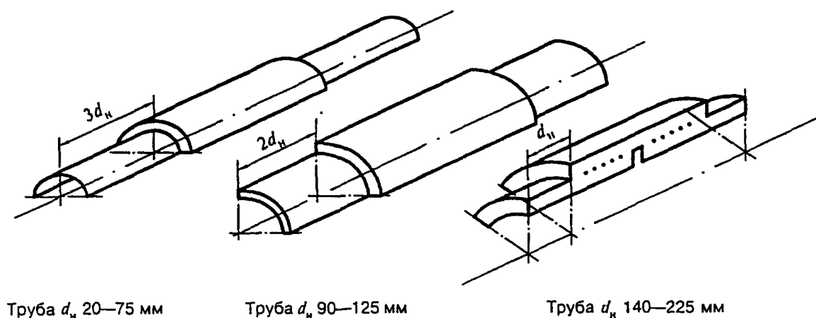
Рисунок Т.1. Общий вид образцов-сегментов
