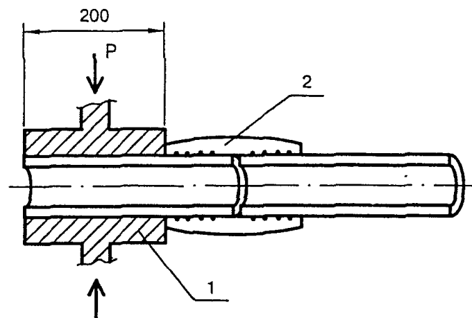
1 - обжимные плиты; 2 - испытываемый образец
