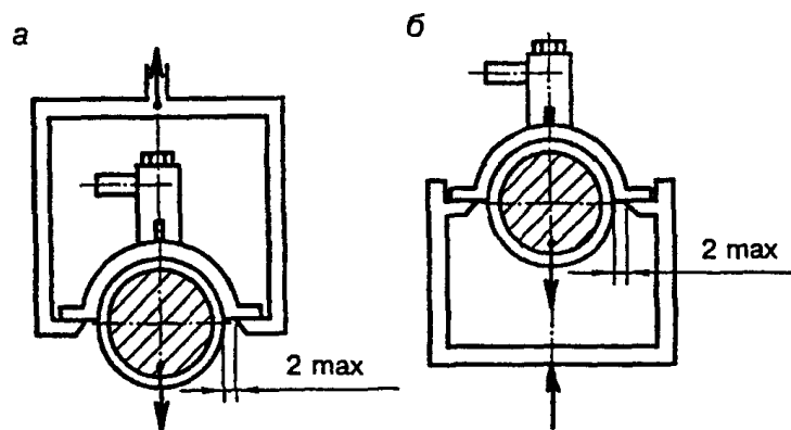
а - отрыв при растяжении; б - отрыв при сжатии
