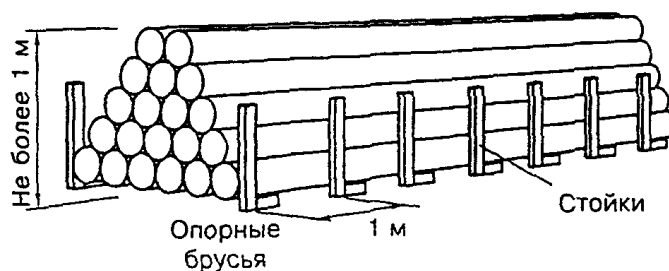
Рисунок 9. Хранение отдельных труб в штабеле
