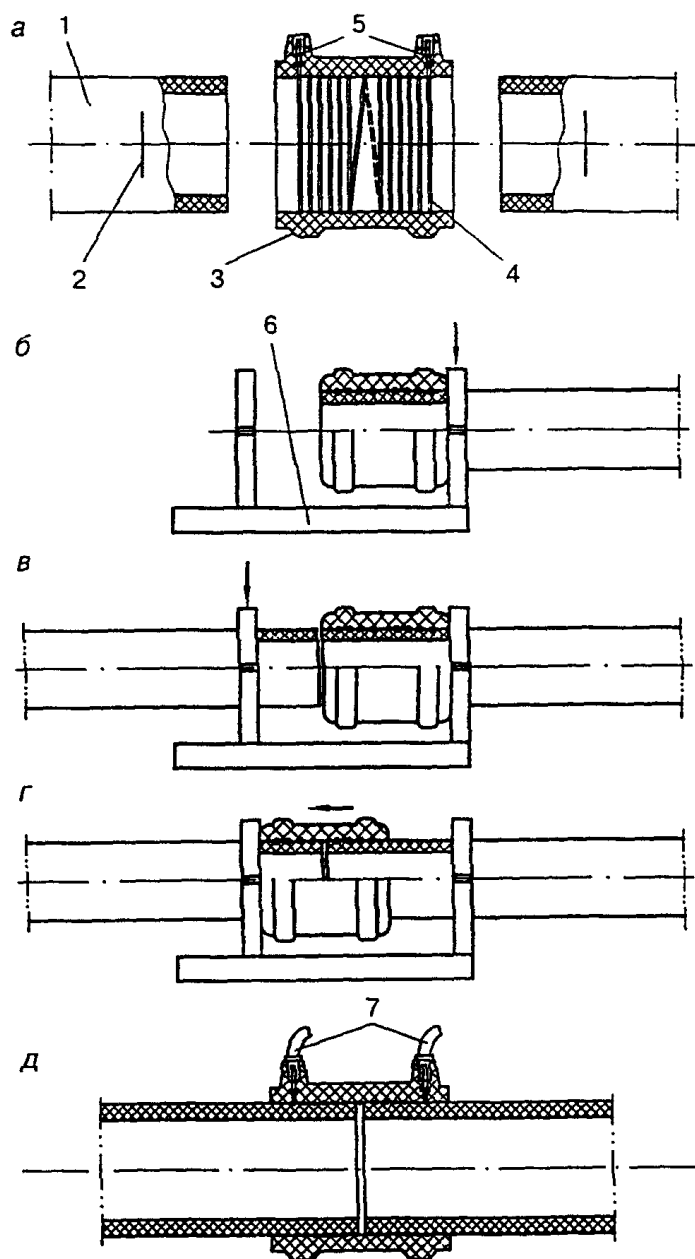
а - подготовка соединяемых элементов; б, в, г - этапы сборки стыка; д - собранный под сварку стык; 1 - труба; 2 - метка посадки муфты и механической обработки
