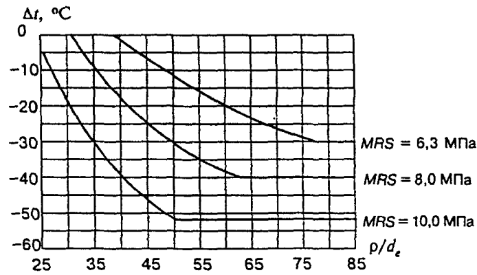
Рисунок 4. Максимально допустимый отрицательный температурный перепад в зависимости от отношения радиуса упругого изгиба к наружному диаметру газопровода при температуре эксплуатации 0 °С и рабочем давлении 0,3 МПа для SDR 11 и различных MRS
