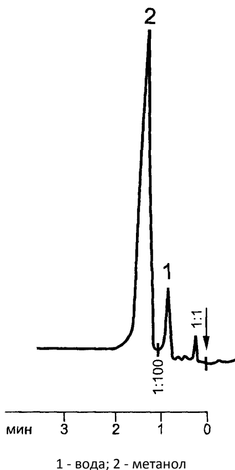
Рисунок Б.1. Типовая хроматограмма технического метанола
