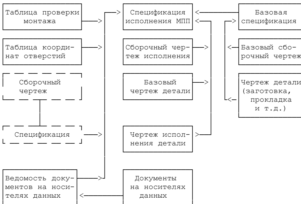
Пример построения комплекта конструкторских документов для МПП
