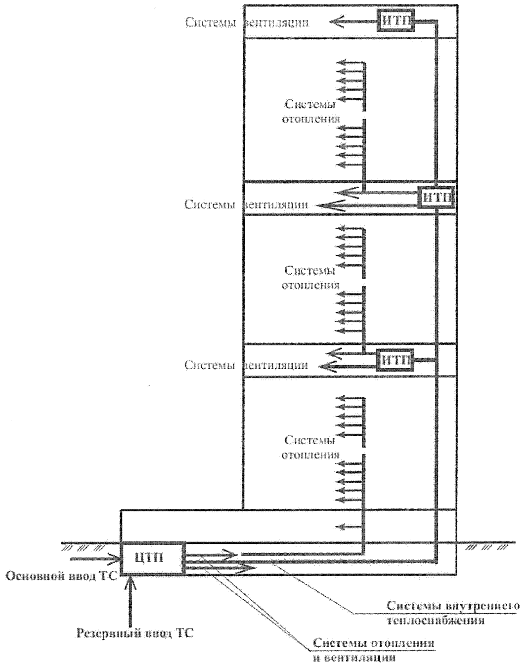
Рисунок 5.1 - Схема теплоснабжения высотного здания от центрального источника
