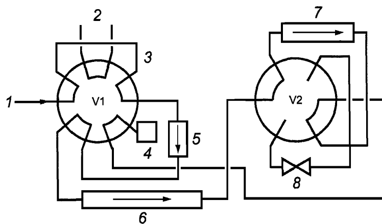
b - Кран 1 (V1) в положении 2 и кран 2 (V2) в положении 1
