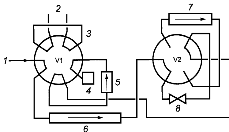
c - Кран 1 (V1) в положении 1 и кран 2 (V2) в положении 2
