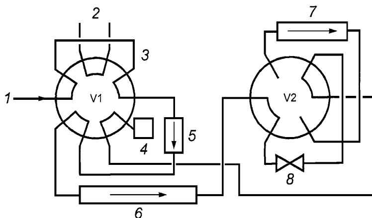
d - Кран 1 (V1) в положении 2 и кран 2 (V2) в положении 2
