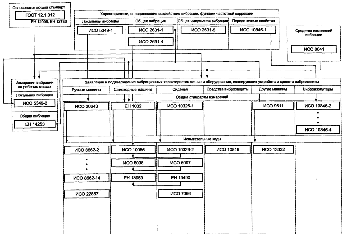
Рисунок Б.1. Схема комплекса международных и европейских стандартов в области вибрационной безопасности
