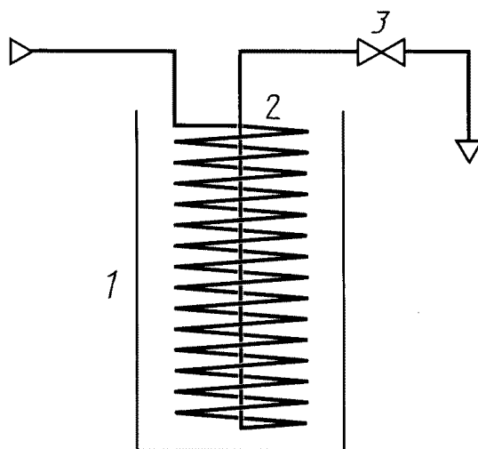
1 - сосуд для охлаждающей смеси; 2 - змеевик; 3 - игольчатый вентиль
