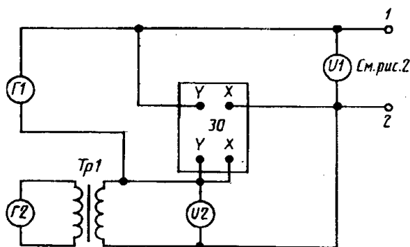
Схема включения аппаратуры для испытания приборов на влияние формы кривой
