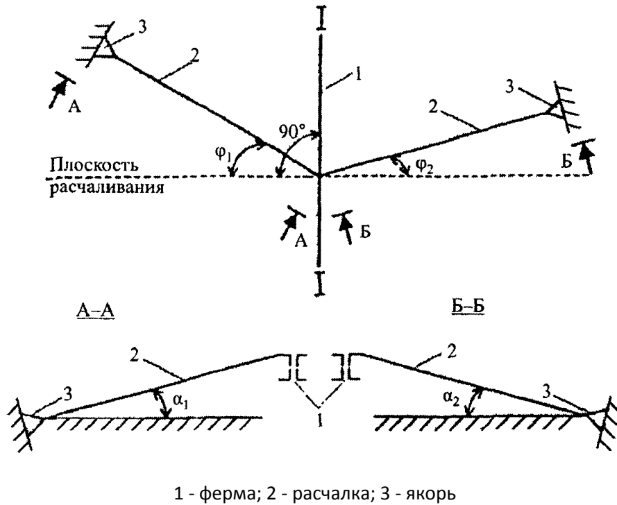
Рисунок К.2. Схема раскрепления ферм расчалками
