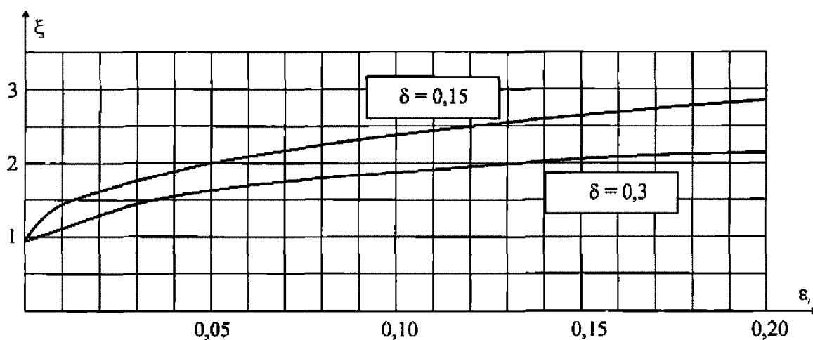
Рисунок 11.1 - Коэффициенты динамичности
