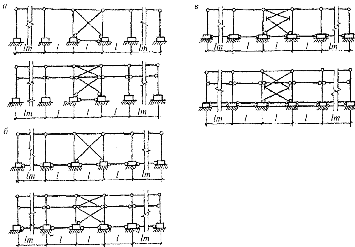
а - в - типы соединений элементов каркаса
