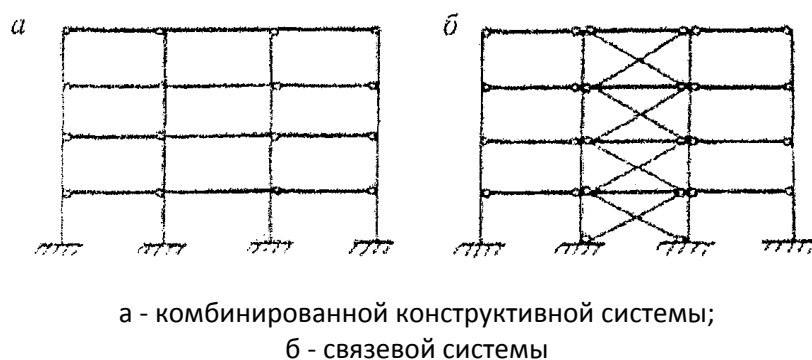
Рисунок В.1. Схемы рам каркасов многоэтажных зданий
