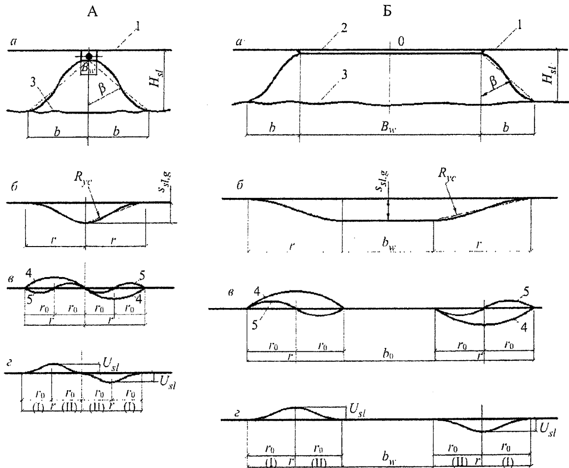
Рисунок 6.1. Схема к расчету просадок основания фундаментов
