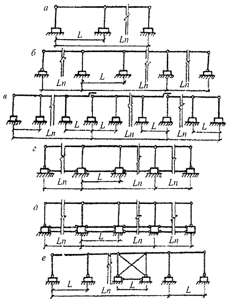
а - е - типы соединений элементов каркаса
