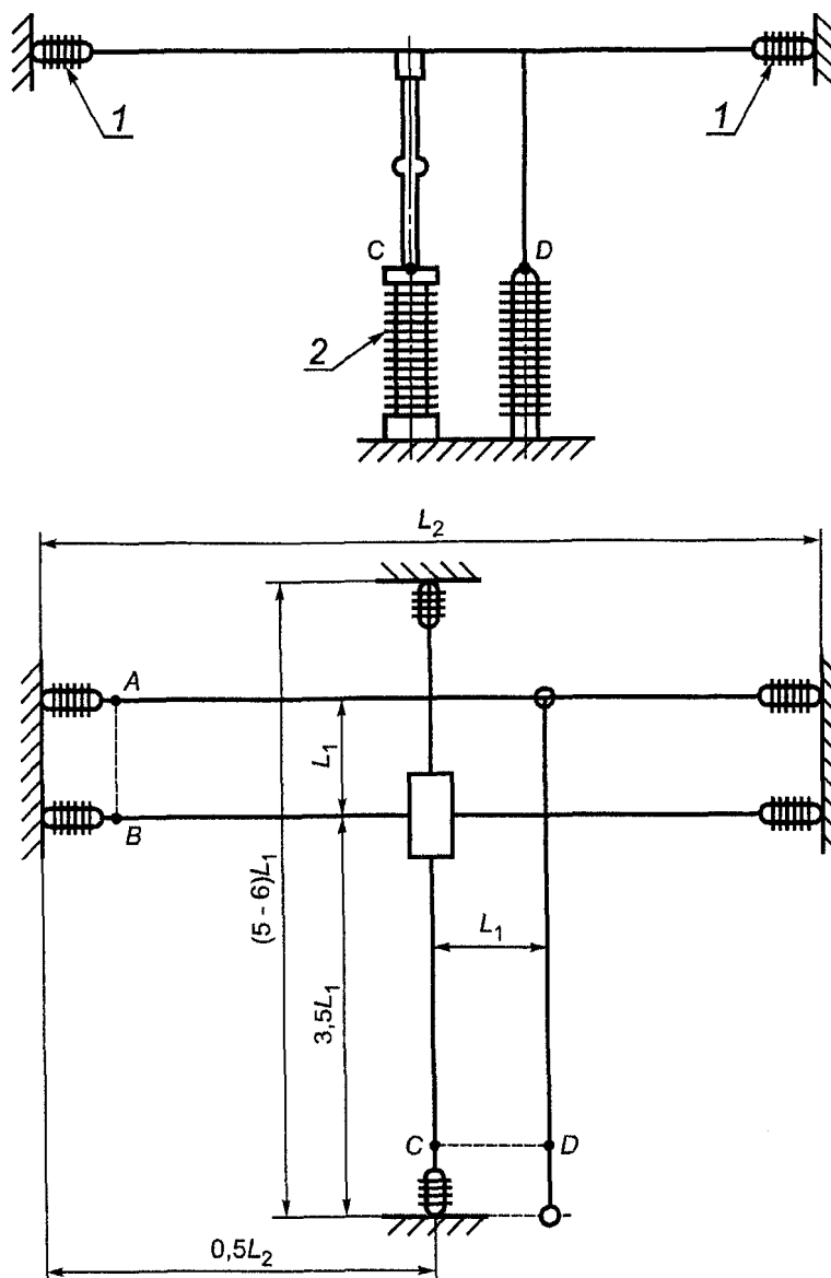
Рисунок 5. Однофазная испытательная установка для разъединителей (заземлителей) с разделенными опорами с вертикальным изолирующим промежутком на номинальное напряжение 110 кВ и выше
