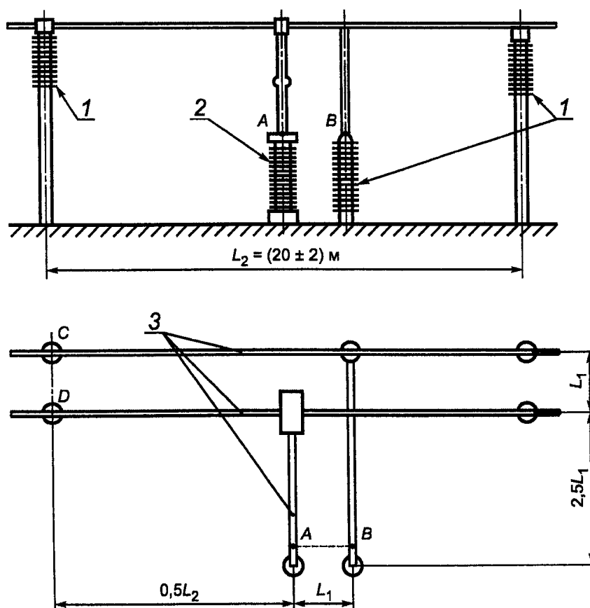
Рисунок 4. Однофазная испытательная установка для разъединителей с горизонтальным изолирующим промежутком и их заземлителей на номинальное напряжение 35 кВ и выше
