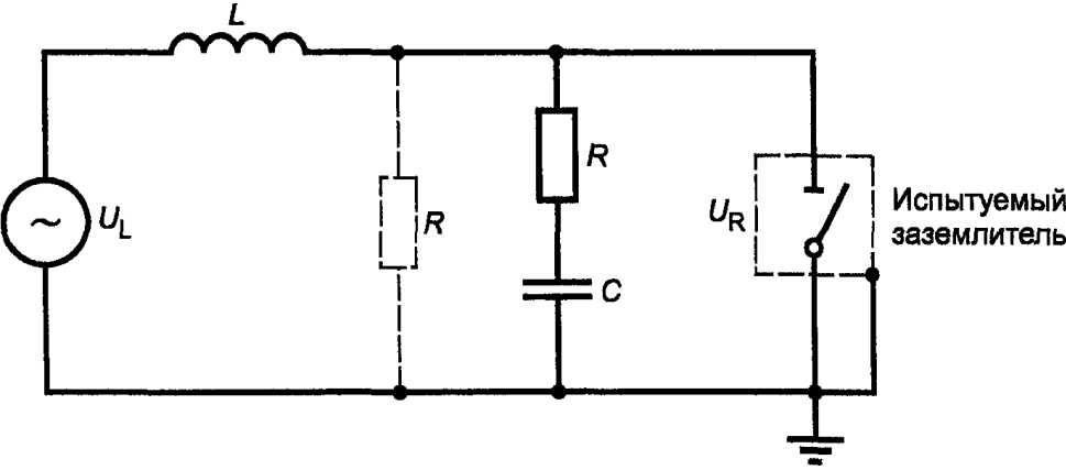
Рисунок 9. Испытательный контур для испытаний на включение и отключение тока, наведенного электромагнитным полем
