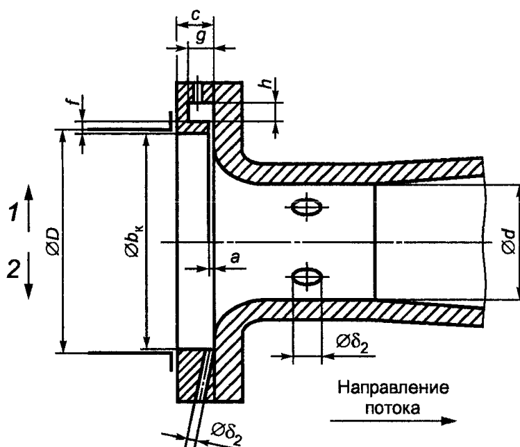
1 - с кольцевой щелью; 2 - с отдельным отверстием
