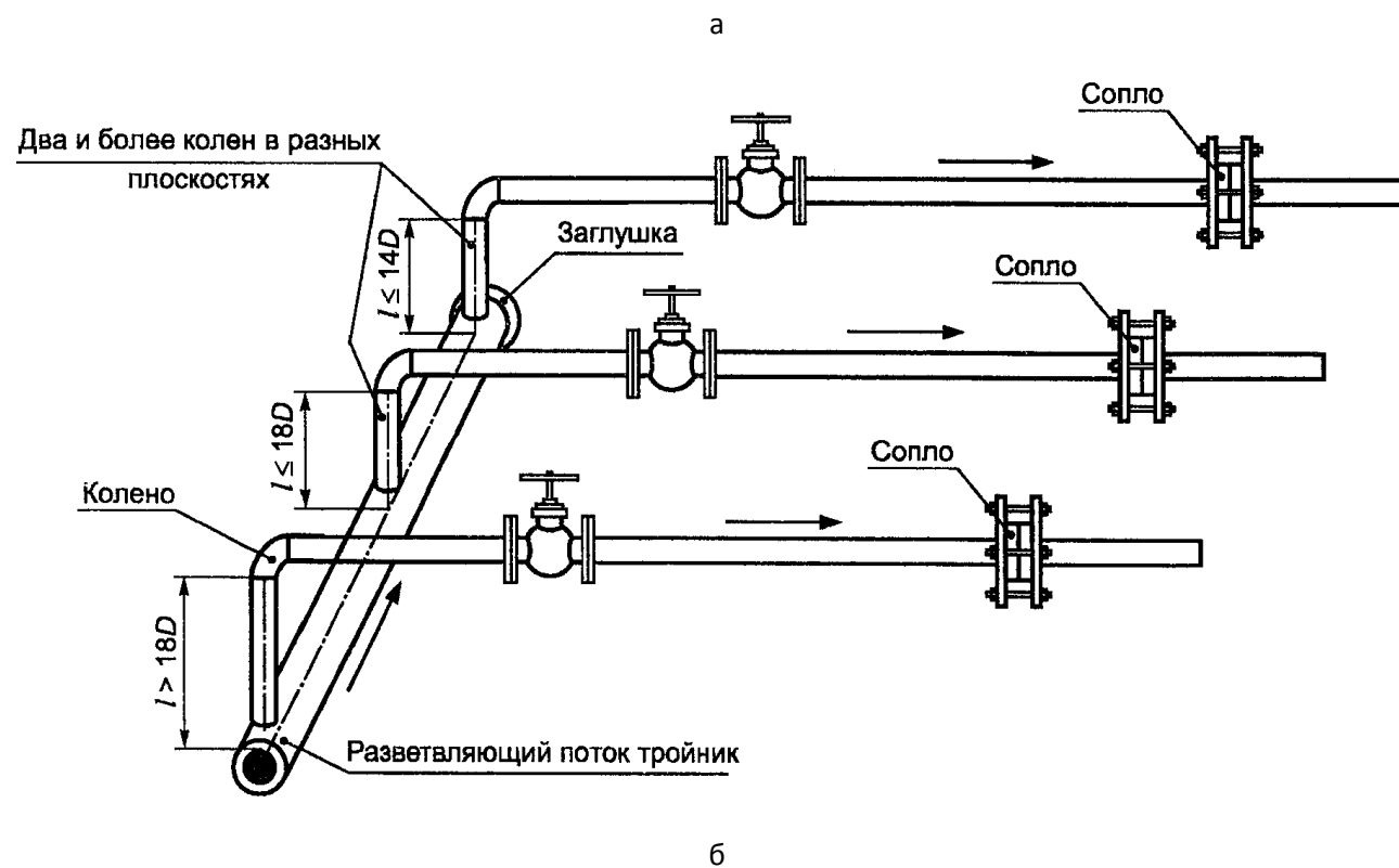
Рисунок 5. Схемы коллектора
