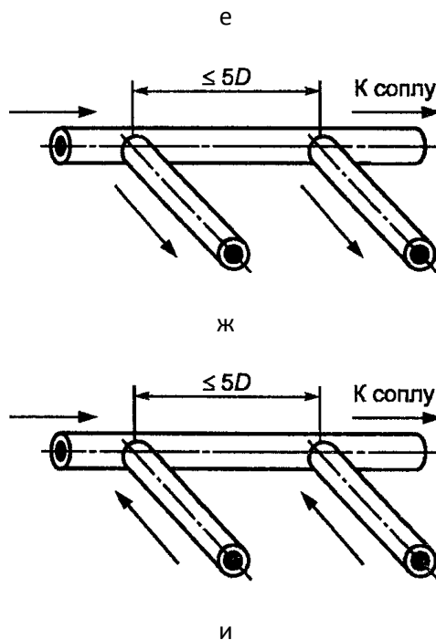
Рисунок А.2. Тройники
