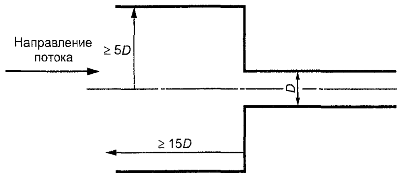
Рисунок А.5. Схема большой емкости
