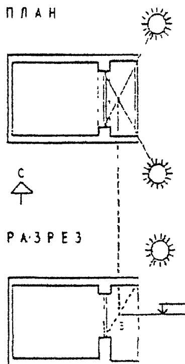
Рис. 3. Схема определения расчетной точки для окна с лоджией.
