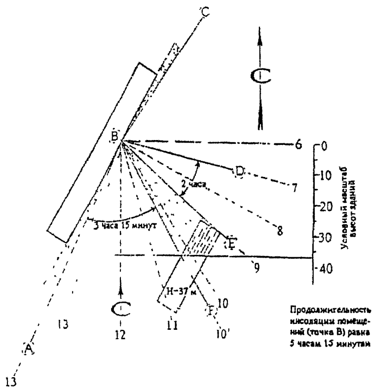
Рис. 5. Схема определения инсоляции.
