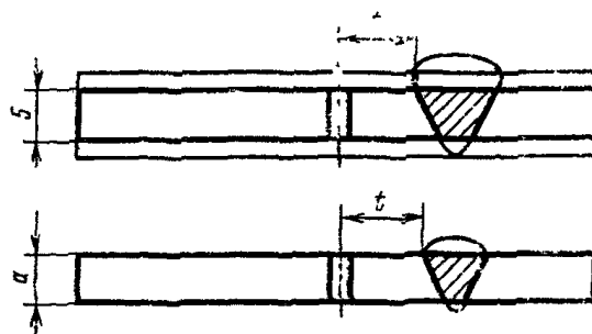
Дуговая сварка
