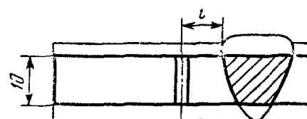
Дуговая сварка
