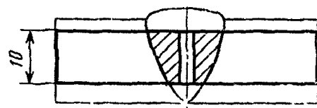
Дуговая сварка 2
