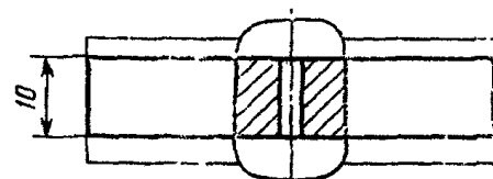
Электрошлаковая сварка и дуговая сварка с принуди- тельным формованием
