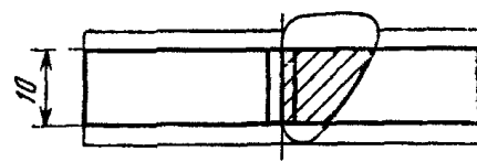
Дуговая сварка по специальной технологии
