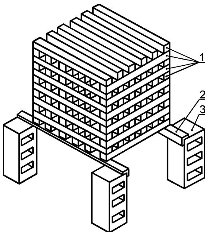
1 - деревянные бруски; 2 - стальной уголок; 3 - бетонный (металлический) блок
