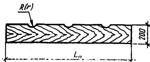
Деревянная подкладка (поз. 3)
