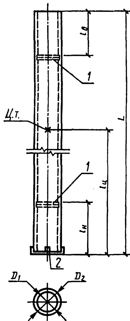
Узлы крепления подпятников
