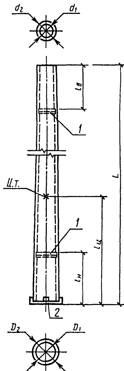
Узлы крепления подпятников
