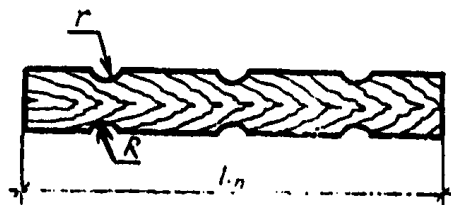
Деревянная подкладка (поз. 3)
