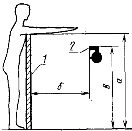
1 - ограждение; 2 - опасный элемент
