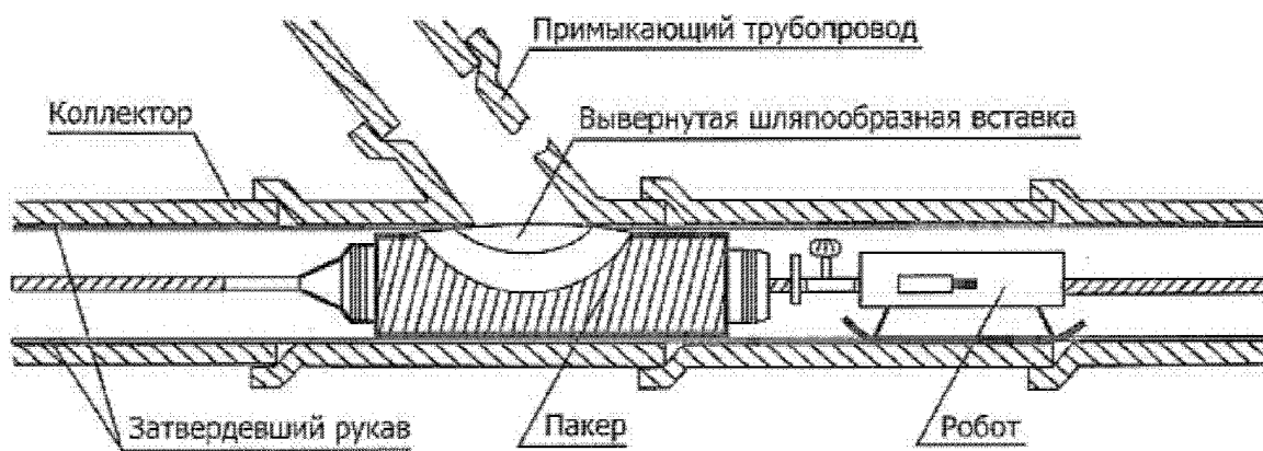
Этап 1. Позиционирование пакера со шляпообразной вставкой
