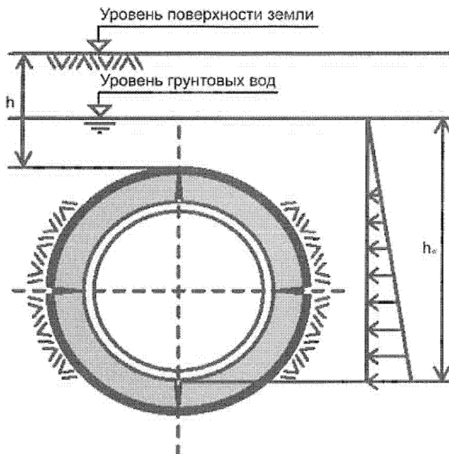
Рисунок 3 - Система "старая труба-грунт". Класс состояния 2
