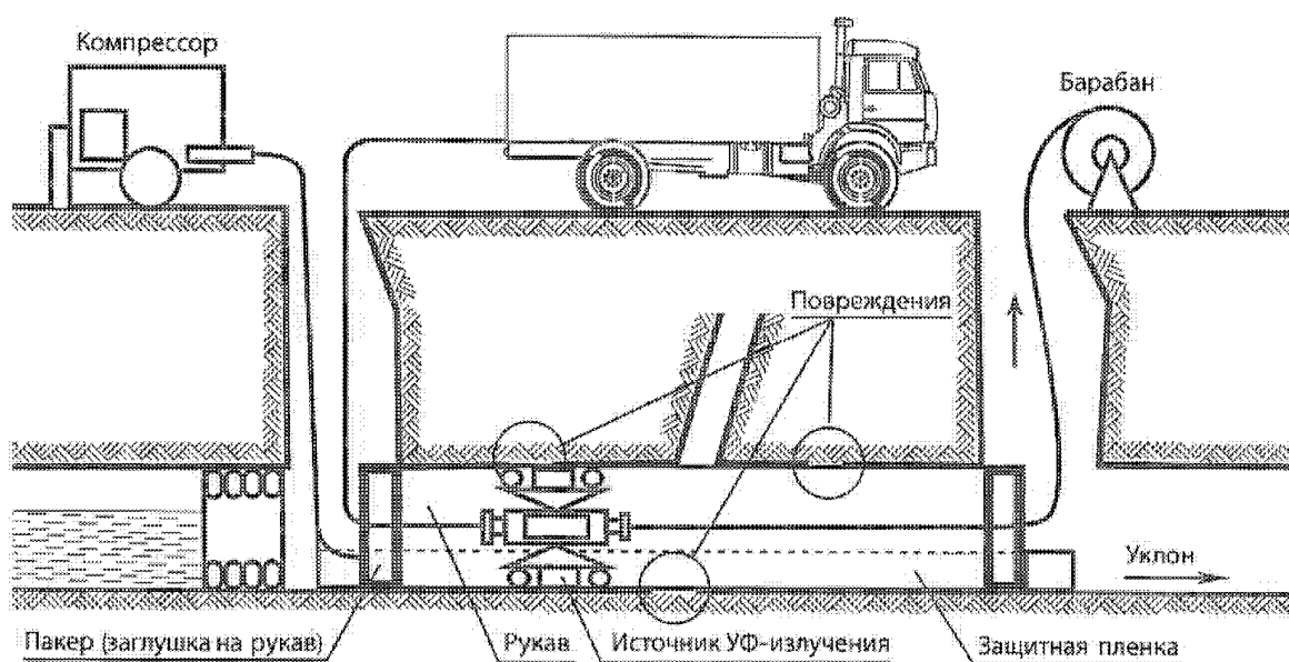
Рисунок 12 - Монтаж гибких полимерных рукавов, отверждаемых УФ-излучением. Позиционирование рукава с помощью сжатого воздуха
