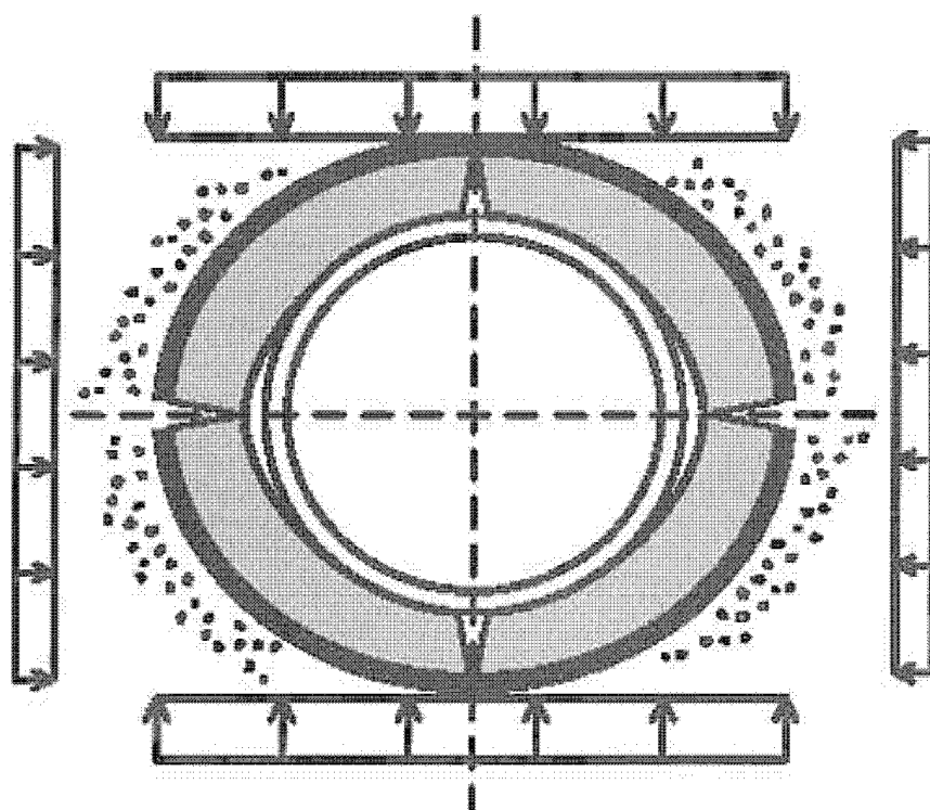
Рисунок 4 - Система "старая труба-грунт". Класс состояния 3
