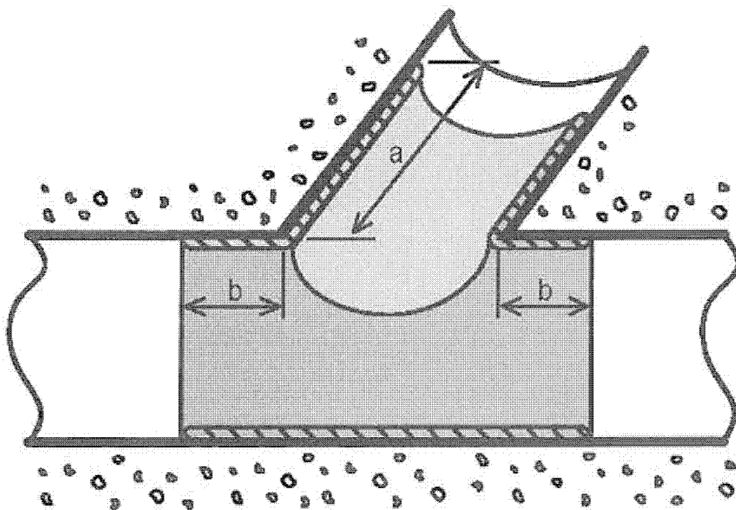
Рисунок 20 - Т-образная манжета
