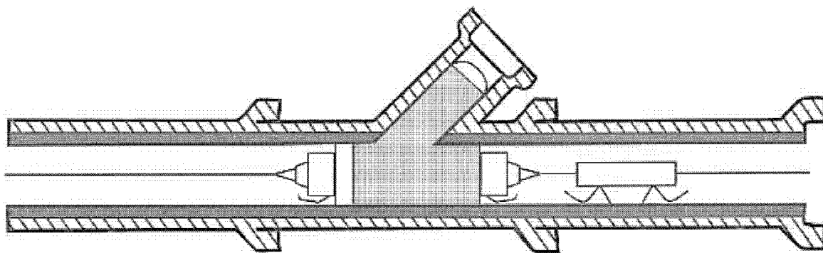
Этап 2. Позиционирование манжеты и ее затверждение
