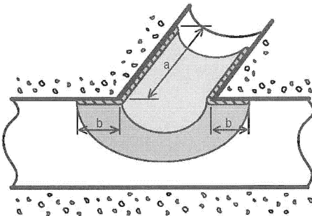
Рисунок 19 - Шляпообразная вставка
