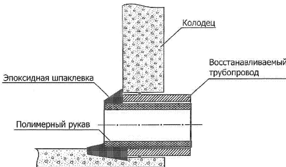
Рисунок 21 - Устройство примыкания с применением эпоксидной шпаклевки
