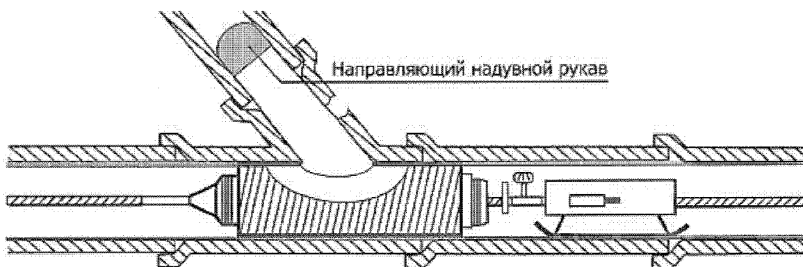
Этап 2. Позиционирование и затвердевание шляпообразной вставки
