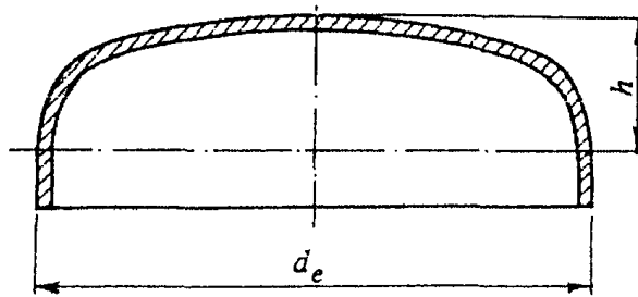
Рисунок А.3. Заглушка эллиптическая
