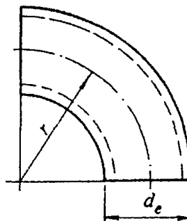
Рисунок А.4. Отвод бесшовный и штамповарной
