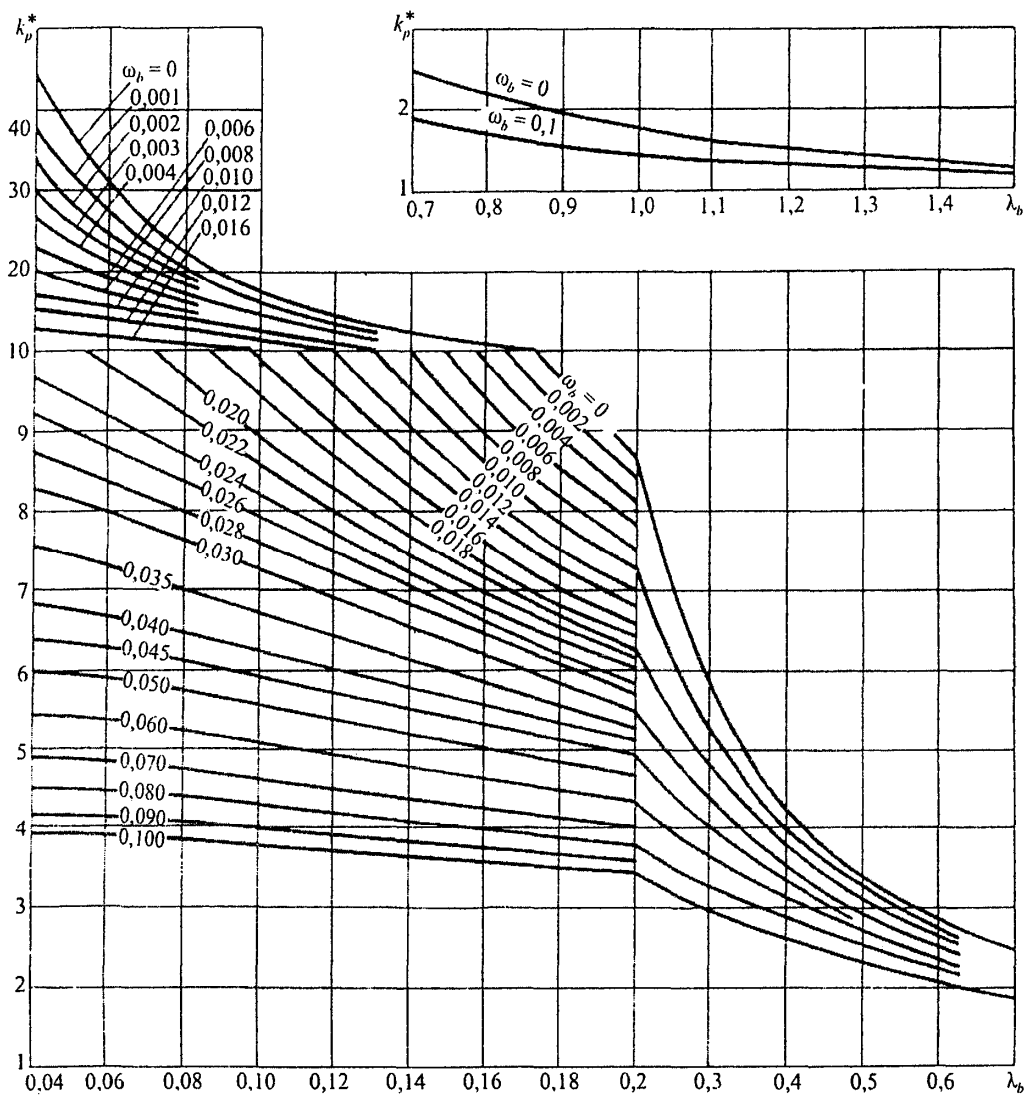
Рисунок 1. График для определения значений коэффициента k_p^*
