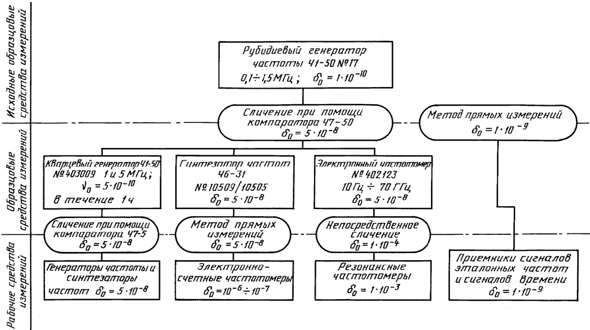
Поверочная схема для средств измерений времени и частоты
